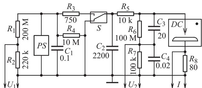
Рис. 1. Принципиальная электрическая схема стенда.
