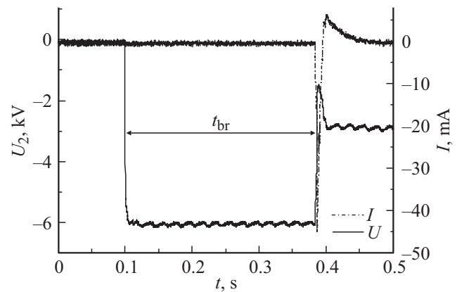
Рис. 2. Осциллограммы напряжения U_2 и тока I разряда при U_1 = -6 кВ.
