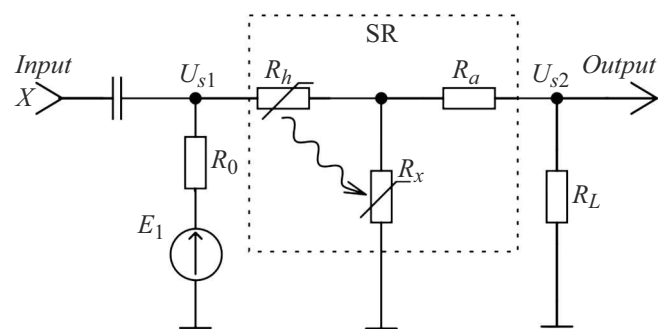
Рис. 3. Схема для измерений параметров синапс-резистора. SR — блок с синапс-резистором. U_{s1} и U_{s2} — напряжения на входе и выходе блока SR соответственно. Резисторы R_h и R_x связаны друг с другом посредством теплопередачи.
