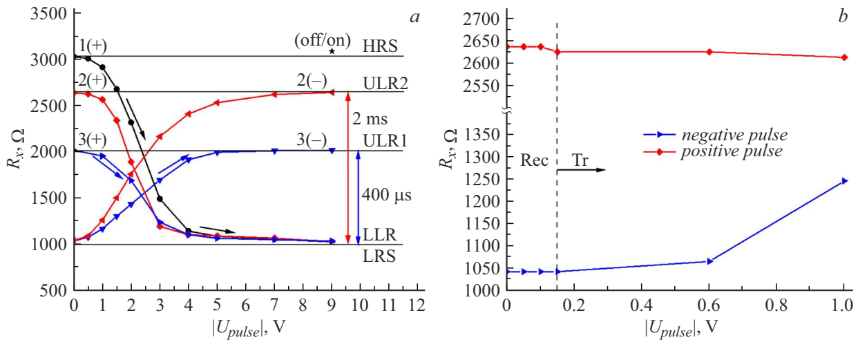
Рис. 5. Зависимость сопротивления синапс-резистора R_x от амплитуды импульсов: a — управляющие импульсы с амплитудой от -9 до +9 V, ULR1 — верхняя граница диапазона сопротивлений синапс-резистора для импульсов длительностью 400 \mu s , ULR2 длительностью 2 ms, LLR — нижняя граница диапазона сопротивлений; b — малые амплитуды импульсов, Rec — режим „распознавание“, Tr — режим „обучение“.
