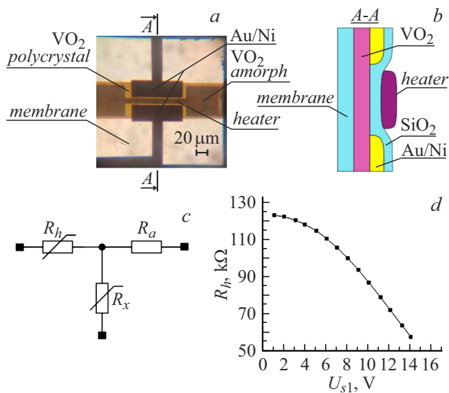
Рис. 2. Конструкция синапс-резистора: a — фотография на просвет синапс-резистора и нагревателя на мембране в оптическом микроскопе; b — схематический рисунок поперечного сечения синапс-резистора и нагревателя; c — электрическая схема соединений: R_h — нагреватель, R_x — синапс-резистор, R_a — дополнительный резистор (на фотографии отсутствует); d — зависимость электрического сопротивления R_h от напряжения U_{s1} .
