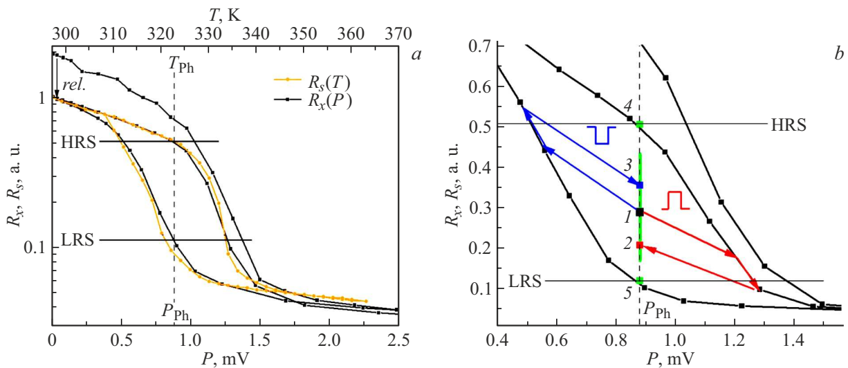
Рис. 4. Диапазон доступных величин сопротивления синапс-резистора: a — сравнение зависимостей R_x(P) и R_s(T) , P — тепловая мощность нагревателя, HRS — состояние с предельно высоким сопротивлением, LRS — состояние с предельно низким сопротивлением, rel — релаксация; b — область фазового перехода, показанная на рис. 4, a , в увеличенном масштабе.
