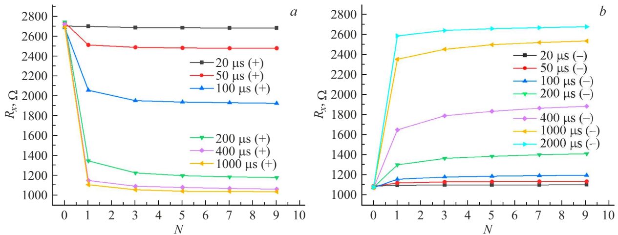
Рис. 6. Зависимость сопротивления синапс-резистора от количества ( N ) поданных импульсов различной длительности: a — исходное состояние ULR, b — LLR (+) — положительные, (–) — отрицательные импульсы.
