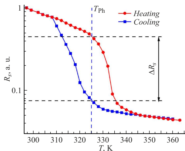
Рис. 1. Зависимость слоевого сопротивления пленки \text{VO}_2 на мембране от температуры R_s(T) . T_{Ph} — температура фазового перехода ПМ. \Delta R_s — диапазон возможных величин слоевого сопротивления при температуре ФП.
