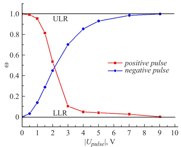
Рис. 7. Зависимость коэффициента связи синапс-резистора \omega от амплитуды управляющих импульсов U_{pulse} .
