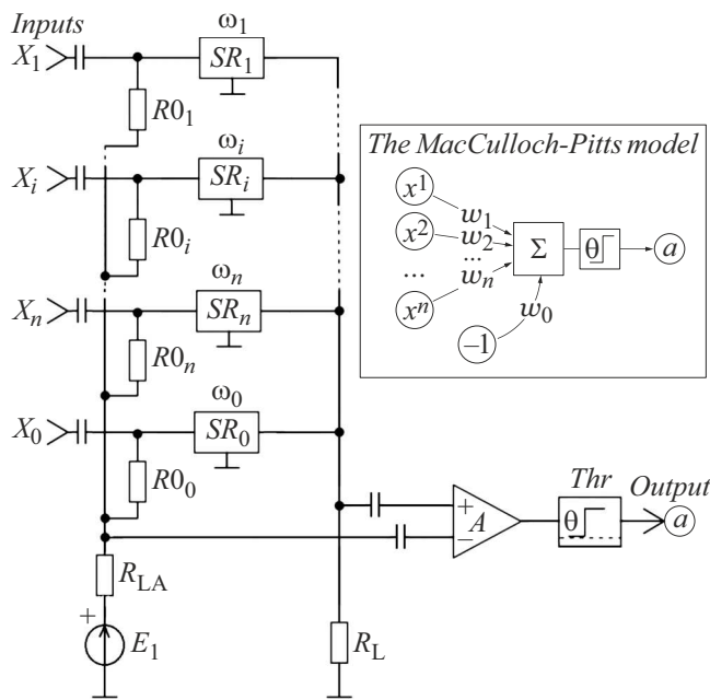
Рис. 8. Искусственный нейрон на основе блоков: SR_1, \dots, SR_i, \dots, SR_n, SR_0 с синапс-резисторами. R_{LA} — входной нагрузочный резистор, R_L — выходной нагрузочный резистор, A — дифференциальный усилитель, Thr — пороговое устройство. X_1, \dots, X_i, \dots, X_n — входные сигналы. X_0 — тормозящий сигнал, a — выходной сигнал. Вставка: искусственный нейрон по модели МакКаллока-Питтса [4].
