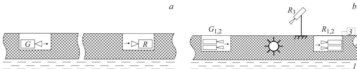
Рис. 4. a — схема эксперимента по радиопросвечиванию ледяного покрова в микроволновом диапазоне: G — генератор, R — многополяризационный радиометр; b — схема выполненного эксперимента просвечивания льда и создания давления в ледяном покрове, инициируемого пороховым зарядом. G_{1,2} — генераторы микроволнового излучения, R_{1,2} — радиометры, 1 — ледяной покров, 2 — вода, 3 — система регистрации, 4 — область подрыва заряда, R_3 — микроволновый радиометр для наблюдения за областью разрушения льда.
