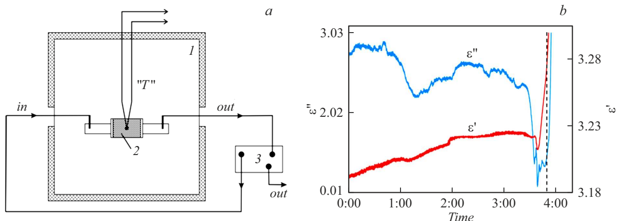
Рис. 1. a — схема экспериментальной установки для исследования диэлектрических характеристик льда: 1 — климатическая камера, 2 — резонатор, 3 — скалярный анализатор, T — датчик температуры; b — зависимость \epsilon' и \epsilon'' льда при его нагревании от времени; измерения вблизи 3.4 GHz; штриховая линия — начало таяния образца при 0 °C.
