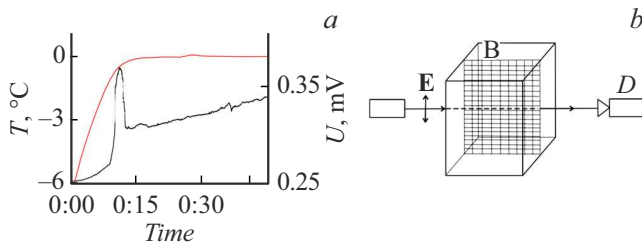
Рис. 6. a — температура льда (верхняя линия) и мощность проходящего линейно поляризованного видимого излучения через образец в зависимости от времени на длине волны 535 nm. Регистрируемая мощность представлена в единицах напряжения фотодетектора ( U ); b — схема расположения параллельных базисных плоскостей ( B — одна из плоскостей) и ориентации вектора электрического поля E .
