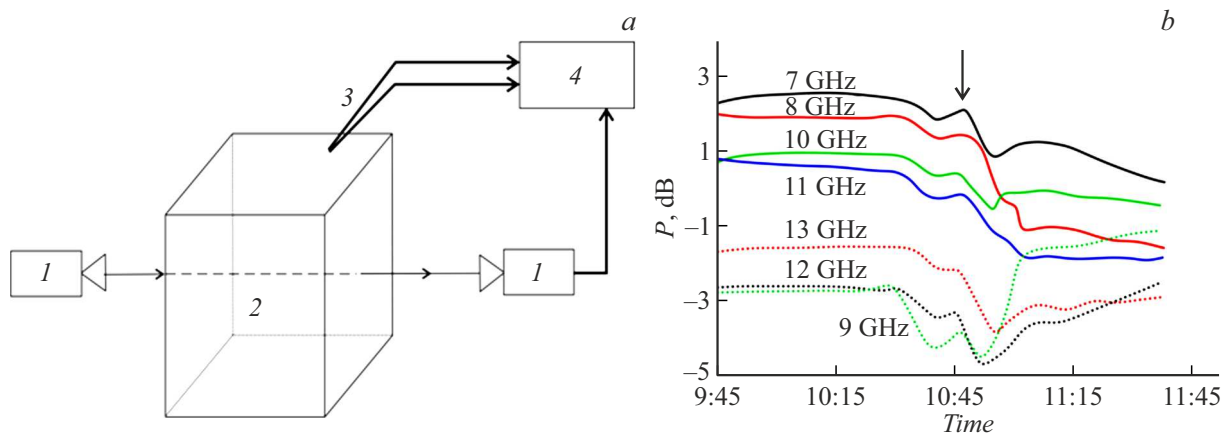
Рис. 2. a — схема установки для измерения мощности ( P ) в децибелах проходящего излучения в микроволновом диапазоне через лед вблизи температуры фазового перехода: 1 — скалярный анализатор цепей, 2 — образец (блок льда), 3 — термопара, 4 — система сбора и записи данных; b — зависимость мощности прошедшего излучения через блок льда на различных частотах от времени. Стрелочкой отмечен эффект „просветления“.
