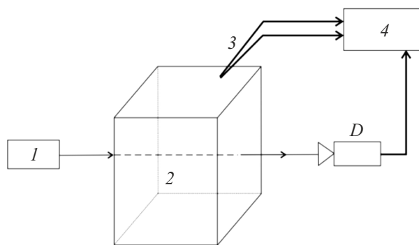
Рис. 5. Схема установки для измерения мощности проходящего излучения в оптическом диапазоне через лед вблизи температуры фазового перехода: 1 — излучатель, 2 — образец (блок льда), 3 — термопара, 4 — система сбора и записи данных, D — фотодетектор.
