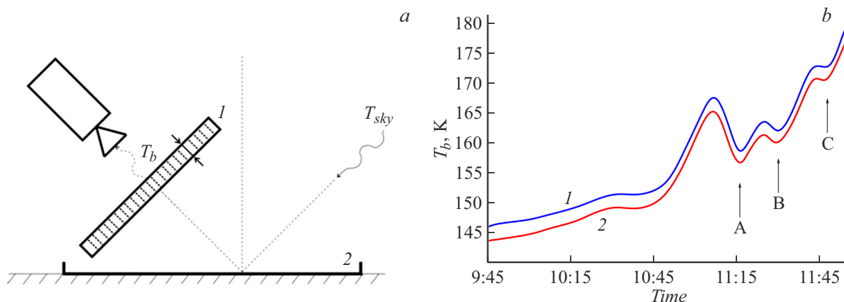
Рис. 3. a — схема экспериментальной установки для исследования теплового излучения образцов льда на фоне холодного неба: R — поляризационный микроволновый радиометр, 1 — плоскопараллельная пластина льда размерами 1000 \times 400 \times 100 mm, T_{sky} — радиояркая температура неба, 2 — металлический лист; b — результаты изменения радиояркой температуры ( T_b ) образца льда со временем. Цифрой обозначена поляризация: 1 — горизонтальная, 2 — вертикальная. Стрелками отмечены области просветления льда.
