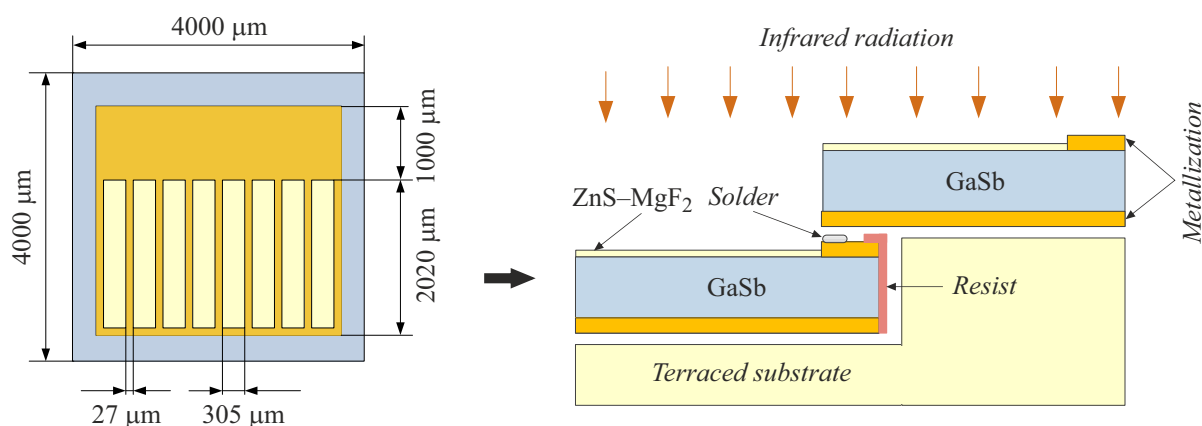
Рис. 1. Соединение двух фотоэлектрических преобразователей за счет перекрытия. На детализации слева — вид освещаемой поверхности ФЭП.
