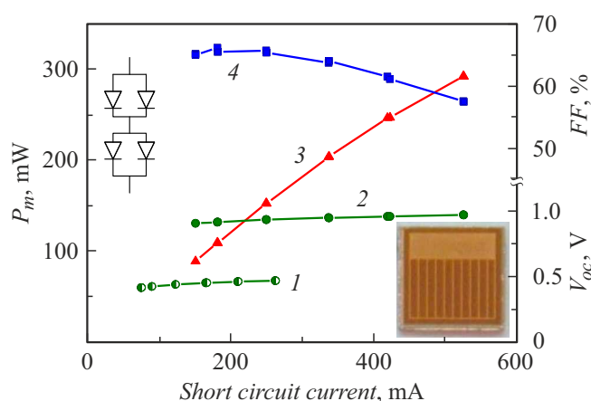
Рис. 3. Электрические параметры преобразователя размером 4 \times 4 \text{ mm} (кривая 1) и модуля (кривые 2–4) террасированного типа с керамическим основанием. 1, 2 — напряжение холостого хода ( V_{oc} ), 3 — мощность в точке оптимальной нагрузки P_m , 4 — коэффициент заполнения ВАХ ( FF ). На вставках — способ коммутации ФЭП в модуле и фотография изготовленного преобразователя.
