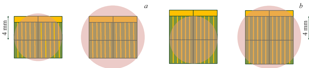
Рис. 4. Потери при облучении модуля ФЭП разной геометрии. a — используемая геометрия (квадратные ФЭП с прямоугольной светочувствительной поверхностью); b — запланированная геометрия (прямоугольные ФЭП с квадратной светочувствительной поверхностью).
