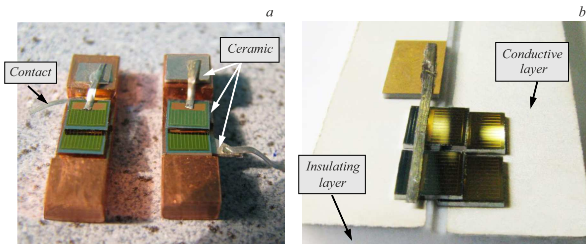
Рис. 2. Соединение преобразователей с односторонней токоотводящей шиной в фотоэлектрический модуль с использованием медного ступенчатого основания (а) и двухуровневой керамической теплоотводящей подложки (b).
