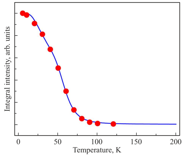
Рис. 3. Температурная зависимость интенсивности люминесценции барьера Cd 0.6 Mg 0.4 Te при ее возбуждении с энергией 2.41 eV при плотности мощности возбуждения W = 5 W/cm 2 . Точки — эксперимент, сплошная кривая — аппроксимация формулой вида (1) с E_{B1} = 0.0065 eV, E_{B2} = 0.046 eV, a_{B1} = 3 и a_{B2} = 12\,000 .
