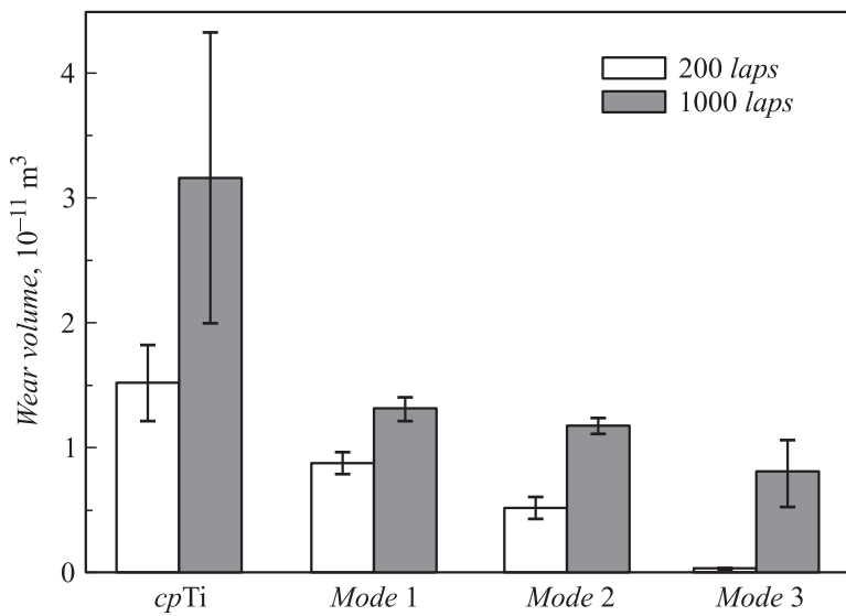
Рис. 3. Объемный износ титана ВТ1-0 и поверхностных сплавов Ti–Al в зависимости от режима синтеза: 1 — \tau \sim 3 \mu\text{s} , 3.5 \text{ J/cm}^2 ; \{[\text{Al}(100 \text{ nm})/\text{Ti}] \times 20\} ; 2 — \tau \sim 3 \mu\text{s} , 3.5 \text{ J/cm}^2 ; \{[\text{Al}(100 \text{ nm})/\text{Ti}] \times 40\} + (\tau = 100 \mu\text{s}, 13 \text{ J/cm}^2, n = 9) ; 3 — \tau = 100 \text{ ns} , 12 \text{ J/cm}^2 ; \{[\text{AL}(1 \mu\text{m})/\text{Ti}] \times 7\} + (50\text{--}100 \mu\text{s}, 11\text{--}12 \text{ J/cm}^2, n = 45) . Контртело: WC–Co.
