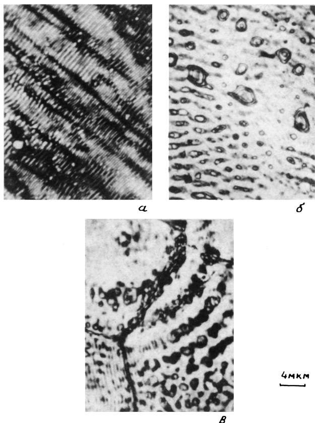
Рис. 1. Структура микрорельефа после лазерного облучения в сплаве Fe-12Cr-Mo-W-V-Nb:
