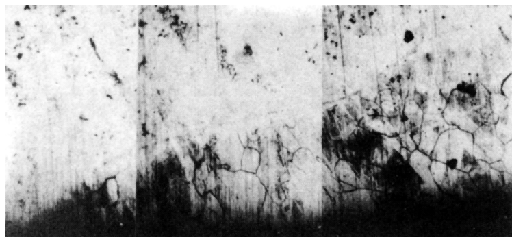
Рис. 4. Структура поврежденного слоя в сплаве Fe-Cr после лазерного облучения.
