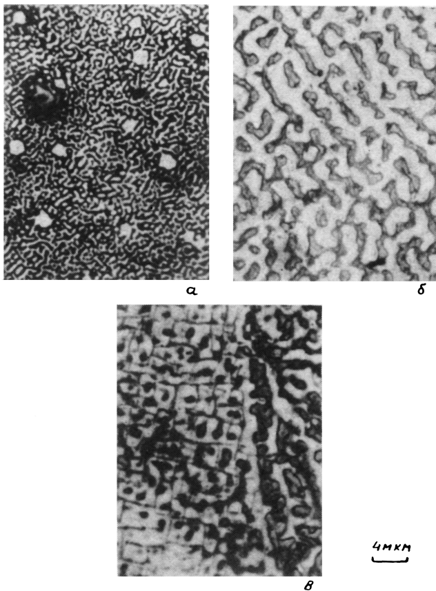
Рис. 2. Структура микро рельефа после лазерного облучения (150 импульсов) в железе (а), сплаве Fe-Cr-Ni (б) и сплаве Fe-Cr (в).
