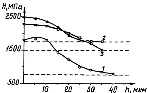
Рис. 3. Изменение микротвердости с глубиной от поверхности в железе (1) и сплавах Fe-Cr (2) и Fe-Cr-Ni (3) после лазерного облучения.
