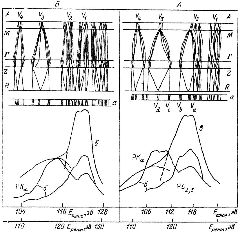
Рис. 7. Структура энергетических зон \text{ZnP}_2(D_4^8) (А) и \text{CdP}_2 (Б), рассчитанная методом псевдопотенциала [13,17], рентгеновские K_\alpha - и L_{2,3} -линии фосфора ( \beta ) [16] и восстановленная L_{2,3} VV оже-линия фосфора в \text{ZnP}_2(D_4^8) и \text{CdP}_2 ( \delta ).
