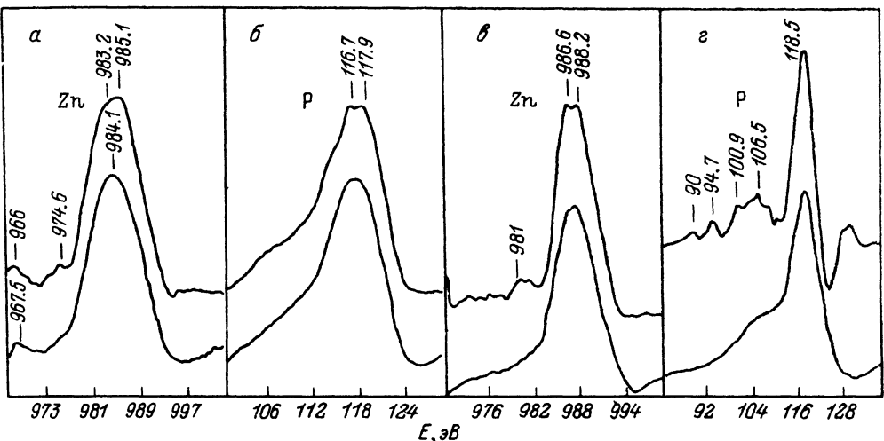
Рис. 4. Исходные и восстановленные оже-линии элементов в соединениях ZnP_2(D_4^8) (а, б) и ZnP_2(C_5^b) (в, г).
