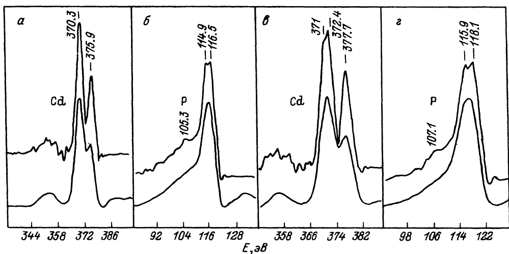
Рис. 5. Исходные и восстановленные оже-линии элементов в соединениях CdP_2 (а, б) и CdP_4 (в, г).
