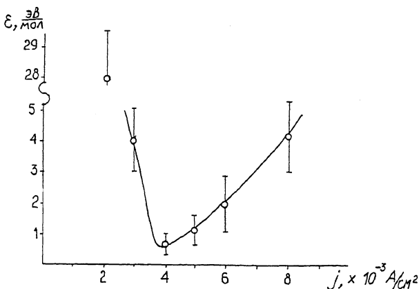
Рис. 2. Энергетическая цена удаления SO_2 в зависимости от плотности тока пучка электронов. Состав смеси: N_2:O_2:H_2O:SO_2 = 84:10:5:1 .
