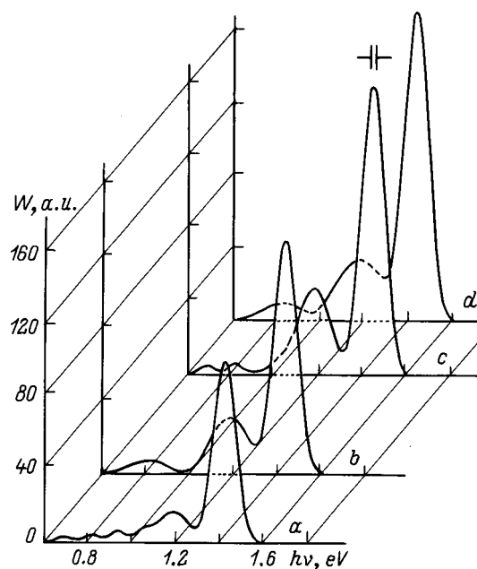
Рис. 4. Спектры фотолуминесценции образцов в n\text{-InP} (111): a — исходный; b-d — после СВЧ облучения в течение 10, 30, 40 s.
