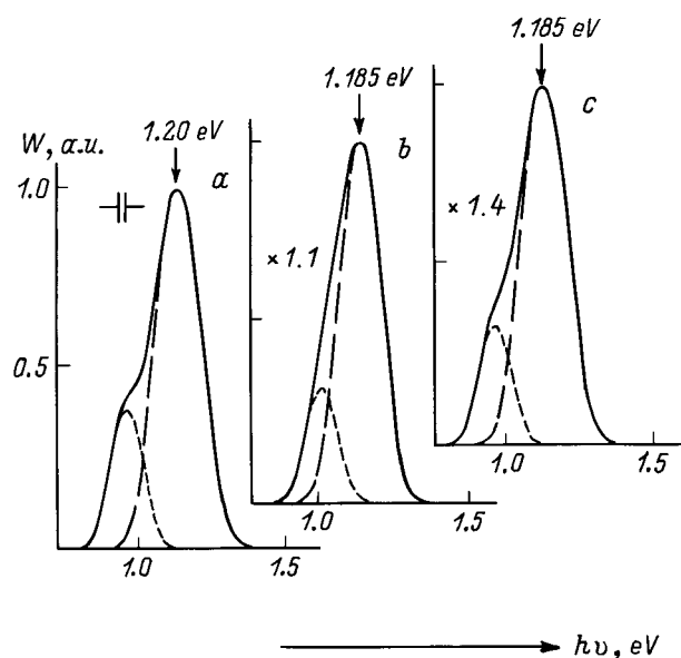
Рис. 3. Спектры фотолуминесценции образцов n\text{-GaAs}:\text{Sn} : a — исходный; b, c — после СВЧ облучения в течение 6 (62) s.
