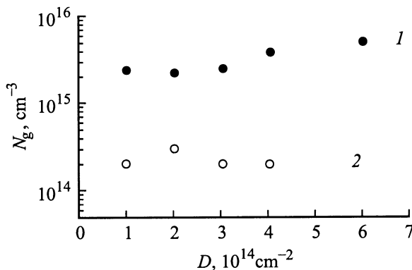
Рис. 5. Зависимость концентрации центров E_c - 0.5 эВ (1) и E_c - (0.16-0.2) эВ (2) после облучения.
