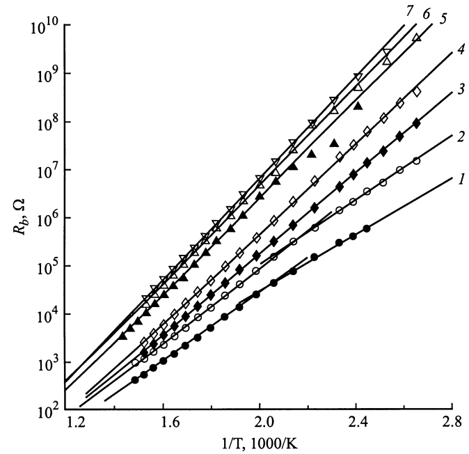
Рис. 3. Температурные зависимости прямого сопротивления диода Шоттки при дозах облучения, 10^{14} \text{ см}^{-2} : 1 — 3, 2 — 4, 3 — 6, 4 — 10, 5 — 20, 6 — 50, 7 — 100.
