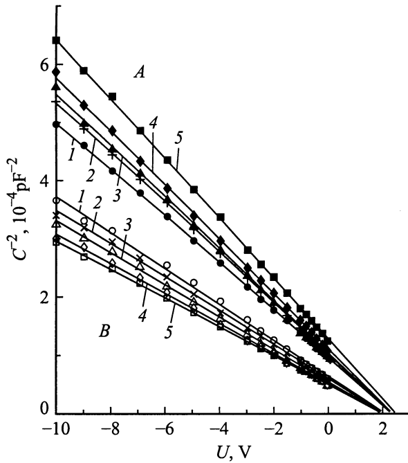
Рис. 1. Вольт-фарадные характеристики p-n -структуры на основе 6H-SiC , измеренные при температурах 300 (серия А) и 650 К (серия В) после облучения дозами, 10^{14} \text{ см}^{-2} : 1 — 1.1, 2 — 2, 3 — 3, 4 — 4, 5 — 6.
