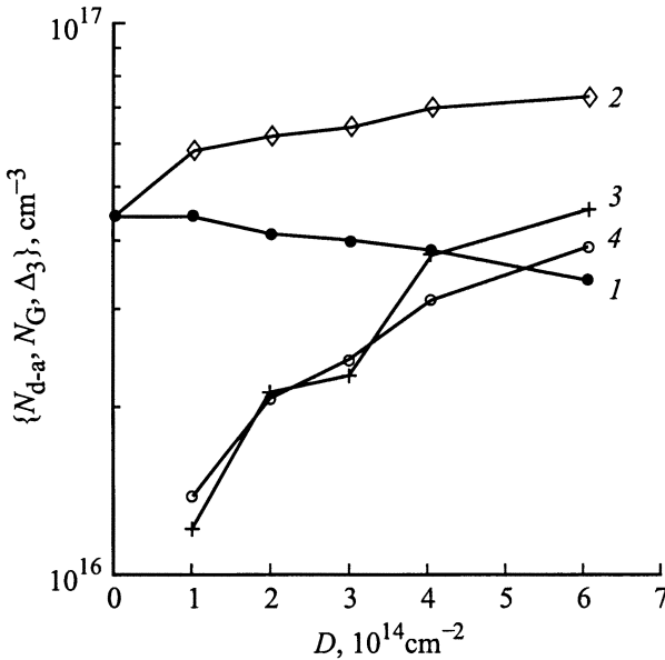
Рис. 2. Зависимость величины N_{d-a} при температурах 300 (1), 650 К (2), их разности \Delta_3 (3) и концентрации центров E_c - (1.1-1.22) \text{ эВ } N_G (4) от дозы облучения.
