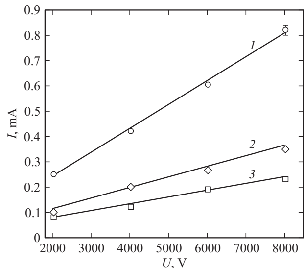
Рис. 3. Контрольные ВАХ источника питания на резисторах: 1 — 1.0, 2 — 3.0 и 3 — 5.0 МΩ.
