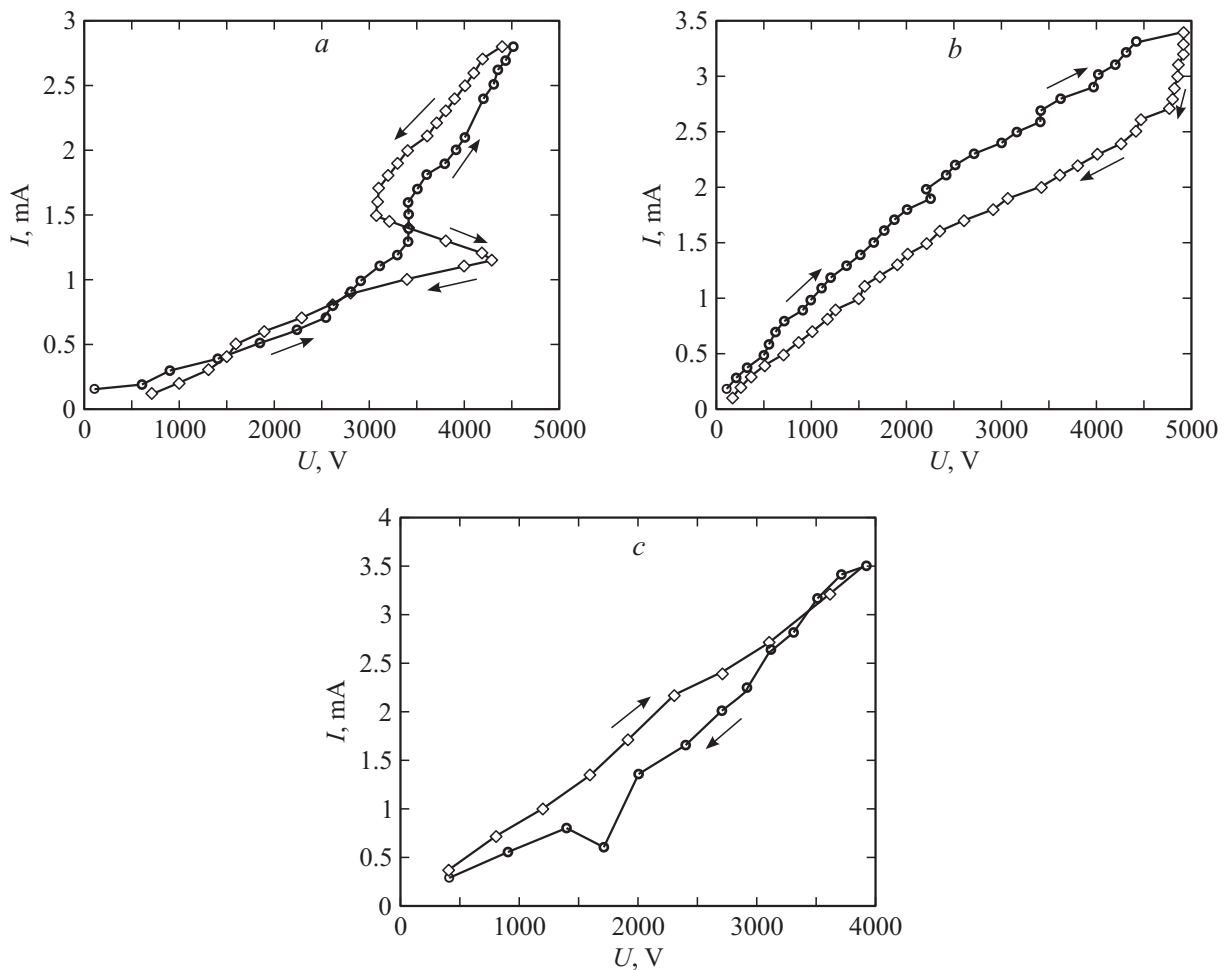
Рис. 4. ВАХ дистиллированной воды, заключенной в стеклянную трубку диаметром: a — 2, b — 4, c — 2–4 mm („усеченный конус“).
