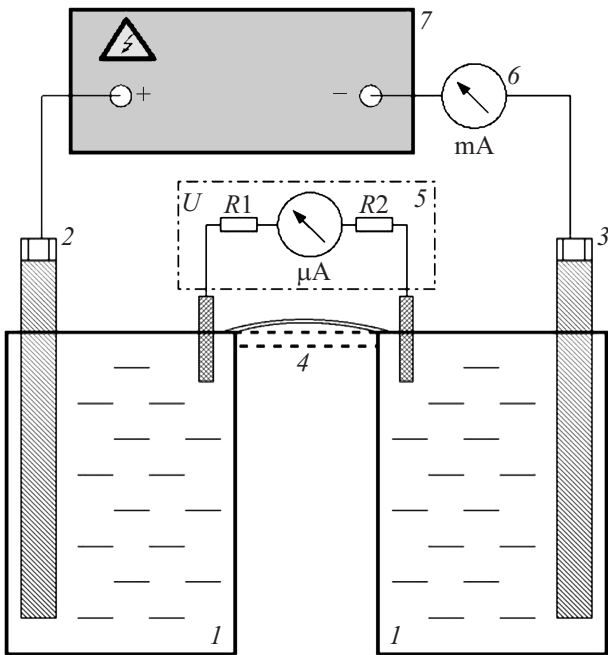
Рис. 1. Схема экспериментальной установки: 1 — сосуды с дистиллированной водой, 2 — анод (нержавеющая сталь), 3 — катод (нержавеющая сталь), 4 — область водного мостика или стеклянной трубки с водой (2–4 мм) с погруженными электродами для измерения разности потенциалов, 5 — высоковольтный вольтметр, 6 — миллиамперметр, 7 — блок регулируемого высокого напряжения (0–30 кВ).
