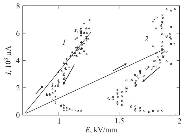
Рис. 2. ВАХ водного мостика (снижение внешнего напряжения). Ограничения по току и напряжению (сверху и снизу) связаны со срывом или пробоем мостика: 1, 2 — разное начальное удельное сопротивление (количество ионов, в том числе примесных) дистиллированной воды. Видны участки отрицательного дифференциального сопротивления (области отрицательного наклона I(U) ).
