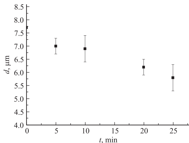
Рис. 3. Зависимость диаметра d пылевых частиц от времени нахождения в плазменно-пылевой ловушке. Условия описаны в тексте.
