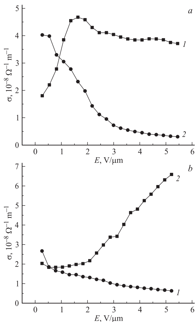
Рис. 6. Зависимость удельной проводимости ячеек хромолан– \text{SiO}_2 ( a ) и хромолан– a -C:H ( b ) от напряженности электрического поля. Кривые 1 — минус на хромолане, 2 — плюс.
