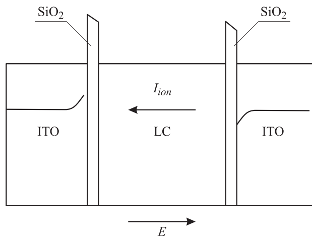
Рис. 4. Схема протекания тока через жидкий кристалл. Оба электрода покрыты слоем кварца.
