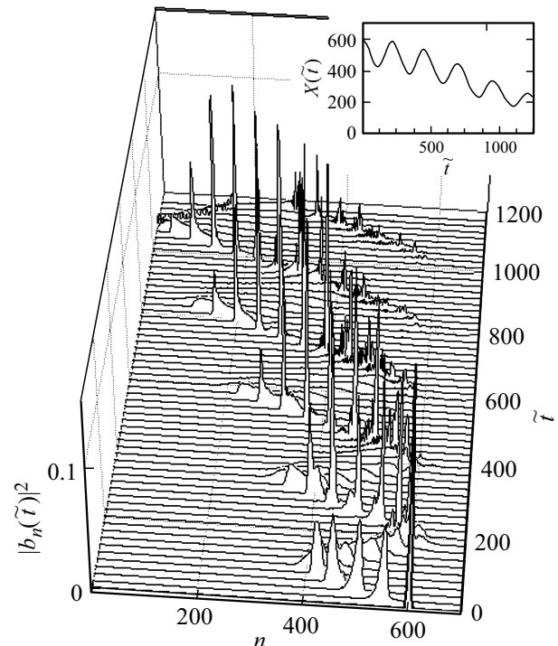
Рис. 7. Графики функций |b_n(\tilde{t})|^2 и X(\tilde{t}) при \kappa = 1 , \eta = 1.276 , \omega = 1 , \omega' = 1 , значение напряженности электрического поля E = 0.03 , для (безразмерного) времени \tilde{t} = 1200 . Длина цепочки N = 701 сайтов.
