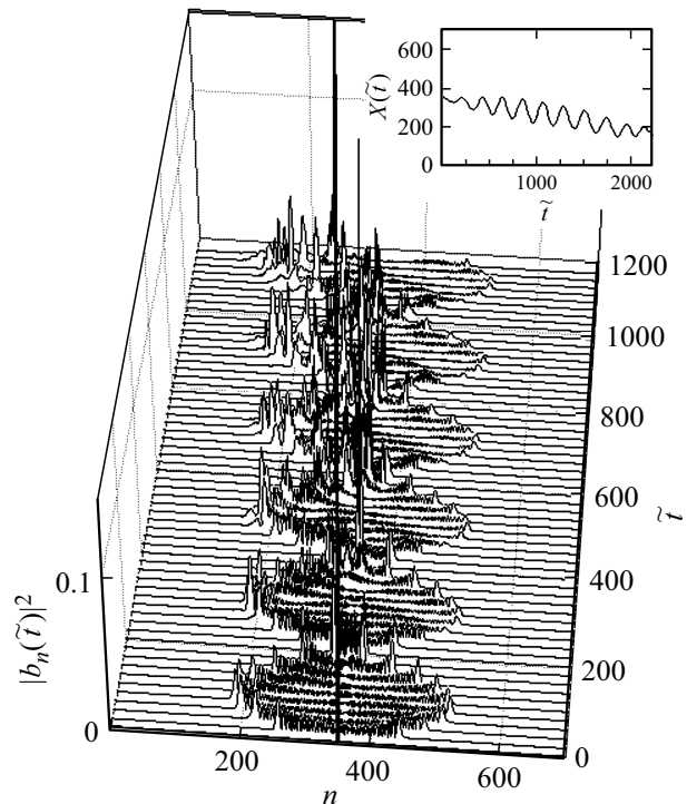
Рис. 9. Графики функции |b_n(\tilde{t})|^2 и X(\tilde{t}) при \kappa = 1, \eta = 1.276, \omega = 1, \omega' = 1 , значение напряженности электрического поля E = 0.03 для (безразмерного) времени \tilde{t} = 1200 . Длина цепочки N = 701 сайтов. В начальный момент времени заряд находится на одном сайте в центре цепочки, u_n^0 = 0 для всех n .
