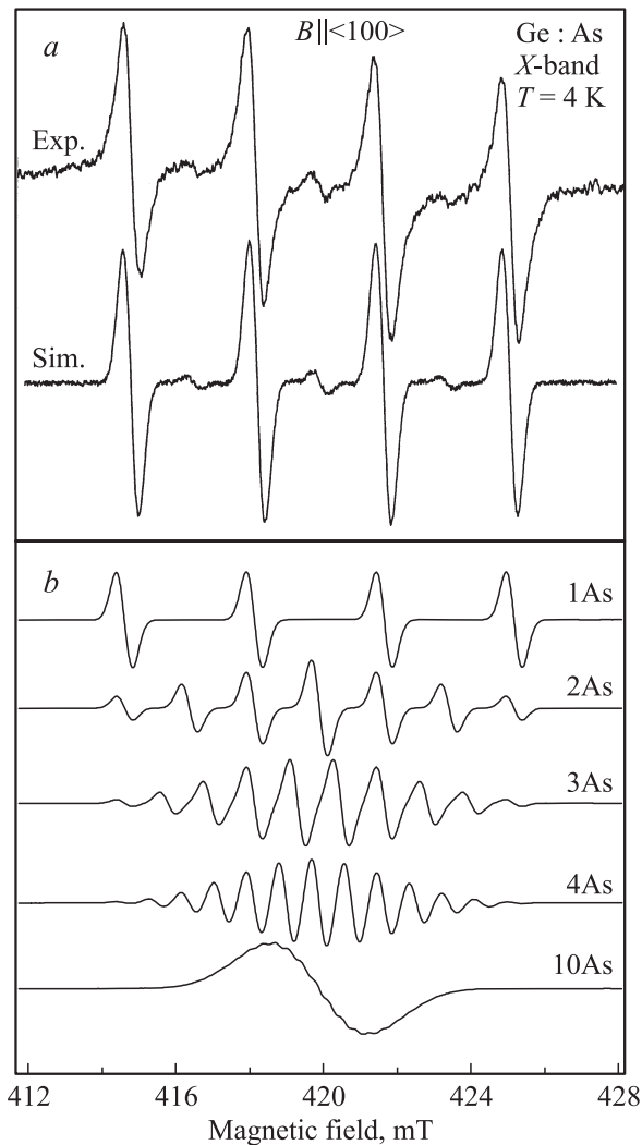
Рис. 2. a ) Спектр ЭПР доноров мышьяка в кристалле германия, обогащенном изотопом ^{74}\text{Ge} (см. таблицу), зарегистрированный при температуре 4 К в ориентации B \parallel \langle 100 \rangle . В нижней части приведен симулированный спектр. b ) Симулированные спектры для одного донора As, а также для обменно-связанных кластеров из двух, трех, четырех и десяти доноров As.
