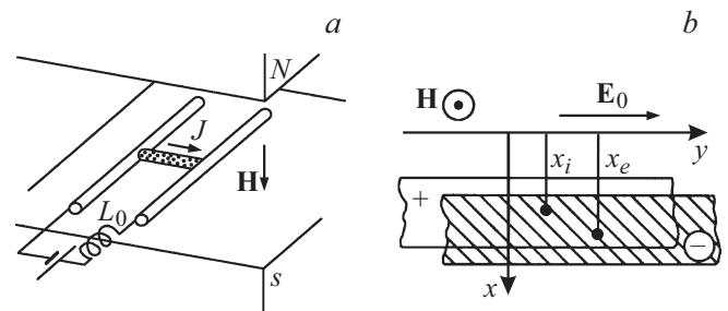
Рис. 2. Схемы рельсотрона (а) и двухблочной модели плазменного ускорителя по А.И. Морозову (б).
