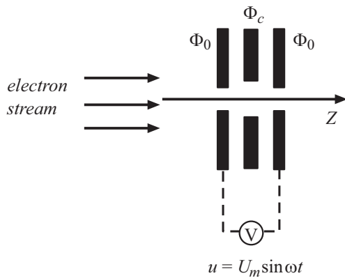
Рис. 1. Трехэлектродная одиночная линза. Переменное напряжение подается к крайним электродам.
