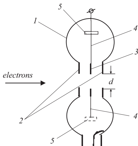
Рис. 2. Тороидальный резонатор с электростатической фокусировкой. Пояснения — в тексте.
