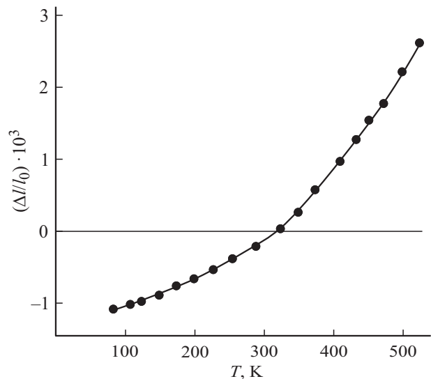
Рис. 4. Температурная зависимость относительного удлинения \Delta l/l_0 монокристаллов \text{FeIn}_2\text{S}_{3.6}\text{Se}_{0.4} .
