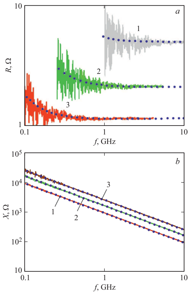
Рис. 2. a — спектры сопротивления R , измеренные антеннами 1–3 при U = 0 . b — спектры реактанса X , измеренные антенной 1 при U = 0 (1), 1.5 (2), 5 V (3). Точки — сглаженные функции R(f) , X(f) .
