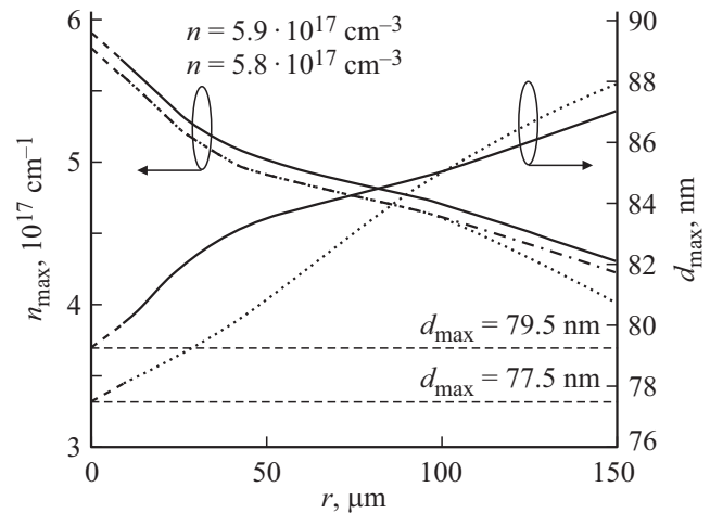
Рис. 2. Зависимость максимального значения в профиле концентрации n_{\max} и координаты d_{\max} , соответствующей максимуму профиля концентрации электронов, от радиуса кругового и ширины кольца кольцевого контактов ( r ) диодов: сплошная линия — до облучения, точечная — после облучения нейтронами 0.5 \cdot 10^{15} см ^{-2} и последующего отжига, штрихпунктирная — аналитический расчет.
