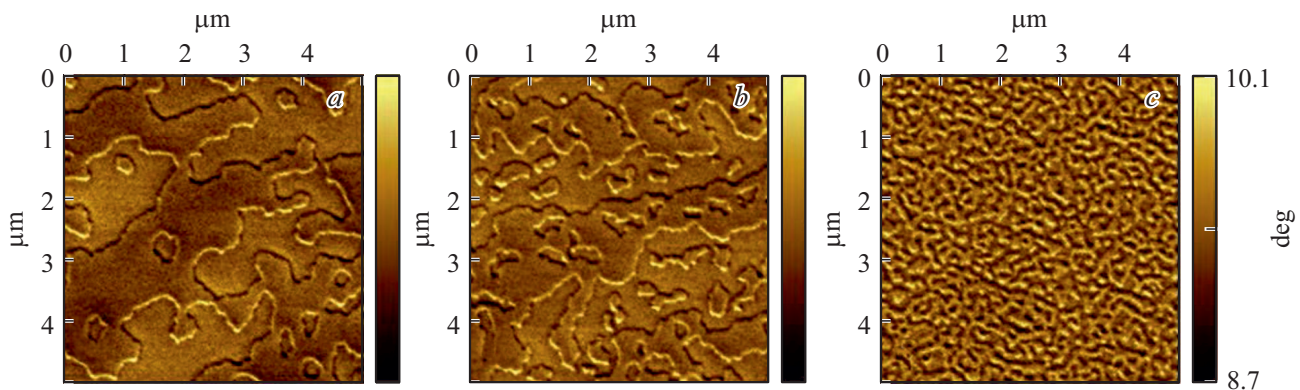
Рис. 4. МСМ-изображения исходной и облученных ионами гелия с различным флюенсом, cm -2 : а — 0, б — 7 \cdot 10^{14} , с — 1 \cdot 10^{15} пленок CoPt(2/5), полученные при сканировании зондом с низким магнитным моментом.
