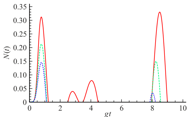
Рис. 2. Отрицательность как функция безразмерного времени gt для сепарабельного начального состояния кубитов |++, +\rangle . Среднее число фотонов в моде \bar{n} = 3 . Безразмерный параметр диполь-дипольного взаимодействия \alpha = 0.75 . Безразмерный параметр керровской нелинейности \chi = 0 (сплошная линия), \chi = 0.2 (штриховая линия) и \chi = 0.3 (точечная линия).
