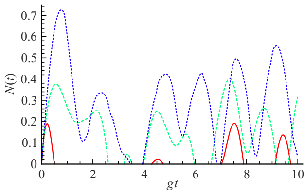
Рис. 1. Отрицательность как функция безразмерного времени gt для сепарабельного начального состояния кубитов |+-, -\rangle . Среднее число фотонов в моде \bar{n} = 3 . Безразмерный параметр диполь-дипольного взаимодействия \alpha = 0.75 . Безразмерный параметр керровской нелинейности \chi = 0 (сплошная линия), \chi = 1 (штриховая линия) и \chi = 3 (точечная линия).
