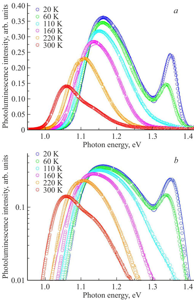
Рис. 1. Спектры ФЛ в линейном (а) и полулогарифмическом (b) масштабах, измеренные в температурном диапазоне 20–300 К (символы — экспериментальные данные, сплошные линии — результат аппроксимации суммой трех гауссовских пиков). (Цветной вариант рисунка представлен в электронной версии статьи).
