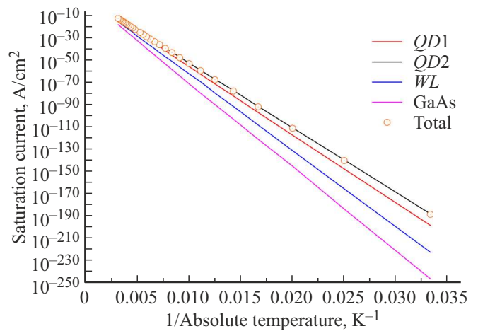
Рис. 3. Температурные зависимости тока насыщения. Линии — различные каналы рекомбинации в GaAs p - n -переходе с \text{Ga}_{0.2}\text{In}_{0.8}\text{As} КТ. Символы — общий ток насыщения.
