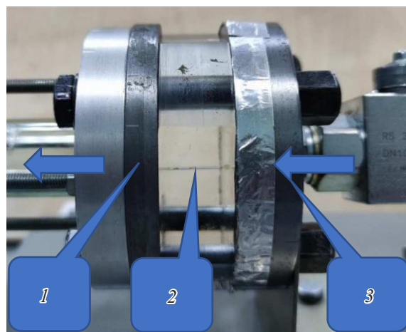
Рис. 1. Конструкция измерительной ячейки. 1 — выходной фланец, 2 — измерительный канал, 3 — входной фланец.
