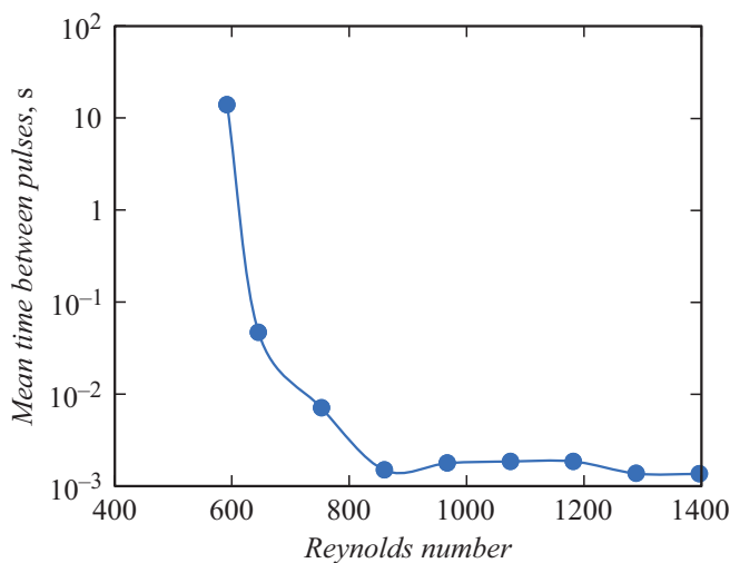
Рис. 2. Средний интервал следования импульсов в зависимости от числа Рейнольдса.
