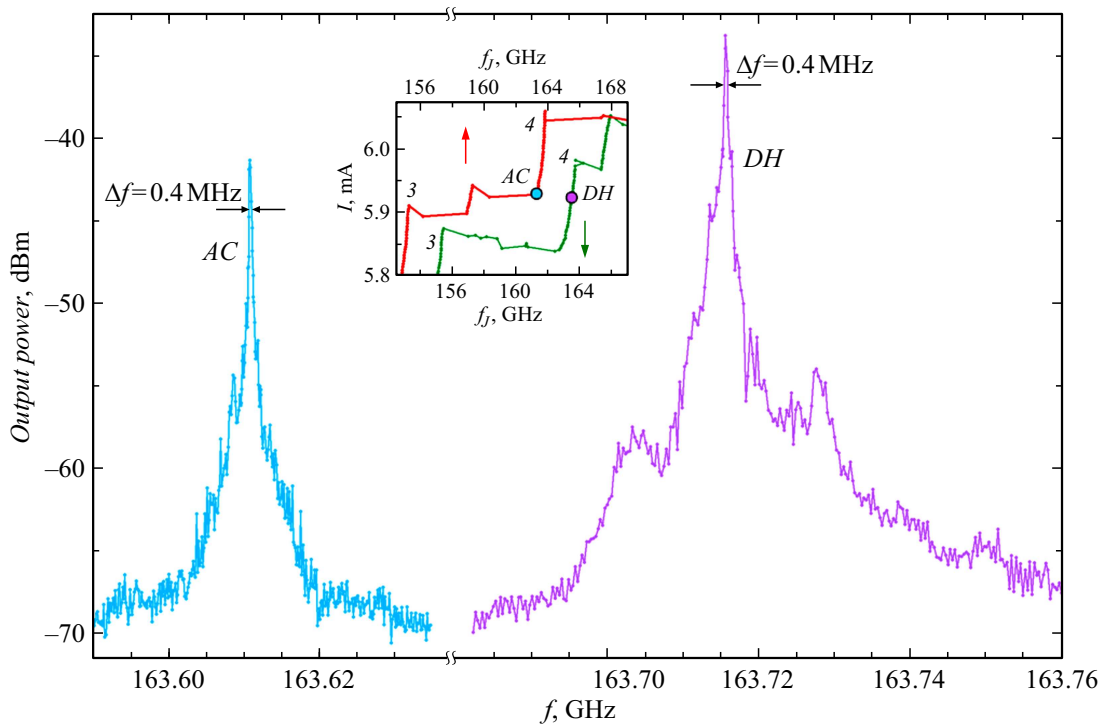
Рис. 5. Спектральные линии джозефсоновского излучения, полученные при подключении к автономному источнику питания двух ( AC ) и четырех ( DH ) секций массива. Гетеродином в измерениях являлась ЛОВ. Линии получены при разрешении анализатора спектра (RBW) 300 kHz. На вставке показаны рабочие точки на ВАХ, в которых наблюдались спектры. Для каждой ВАХ по горизонтальной оси вместо напряжения отложена усредненная джозефсоновская частота.
