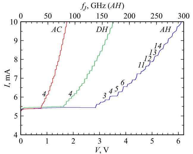
Рис. 3. ВАХ двух ( AC — подключены контактные площадки A и C , см. рис. 1), четырех ( DH ) и всех семи ( AH ) секций массива джозефсоновских контактов. ВАХ получены при увеличении тока смещения (прямые ветви). Верхняя ось обозначает среднюю джозефсоновскую частоту f_J полного массива ( AH ). Для получения f_J частей AC и DH массива необходимо значения на верхней оси умножить соответственно на 7/2 и 7/4. Спектральные измерения проводились на пронумерованных ступенях, нумерация отсчитывается от f_J = 139 GHz — начала резистивной ветви ВАХ массива AH .
