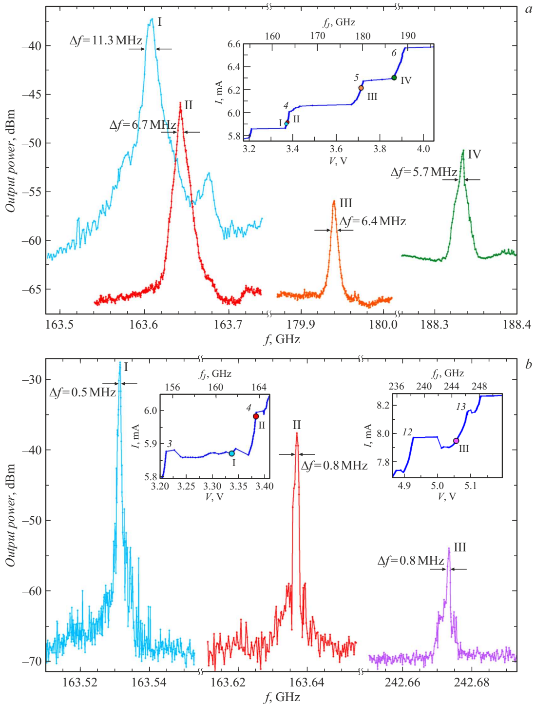
Рис. 4. Спектральные линии джозефсоновского излучения при подключении к массиву источника тока Keithley 6221 (a) и при автономном питании массива (b). Линии I (a, b) получены при использовании в качестве сигнала гетеродина основной гармоники ЛОВ, линия III (b) — при использовании в качестве такого сигнала 2-й гармоники ЛОВ, остальные — когда гетеродином являлся НЧ генератор. Около каждой линии указана ее ширина, измеренная на уровне 1/2 от максимального значения. Линии I и IV (a) получены при разрешении анализатора спектра (RBW) 3 MHz, линии II и III (a) — при разрешении 1 MHz, все линии (b) — при разрешении 300 kHz. На вставках изображены ступени тока ВАХ с отмеченными на них рабочими точками, в которых были получены приведенные спектры. Ступени пронумерованы согласно рис. 3. Искажение ВАХ (b) по сравнению с ВАХ на рис. 3 объясняется выбранной схемой питания массива, при которой на некоторых участках ВАХ не реализуется режим задания тока.
