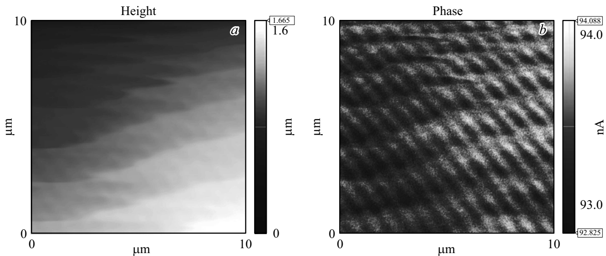
Рис. 2. Результаты магнитно-силовой микроскопии (INTEGRA-AURA (NT-MDT, Россия)): рельеф поверхности (а) и фазовый контраст (b).
