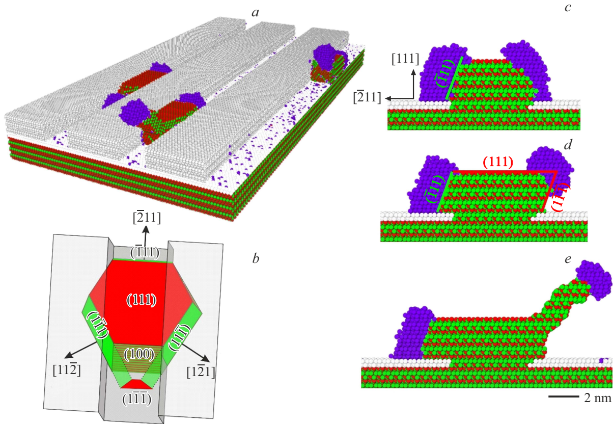
Рис. 2. Кинетика срыва роста НПП. Структурированная подложка с НП GaAs в трех канавках при W = 8 нм (a); схематическое изображение кристалла под каплей в канавке (b); сечения НП во второй канавке в моменты времени t = 0.11 с (c), 0.15 с (d), 0.2 с (e) после начала осаждения Ga и As 2 при F_{Ga} = 1.1 МС/с, F_{As_2} = 11 МС/с, T = 890 К. Фасетки (111)А отмечены красным цветом, а (111)В — зеленым. Ga(I) обозначен фиолетовым цветом.
