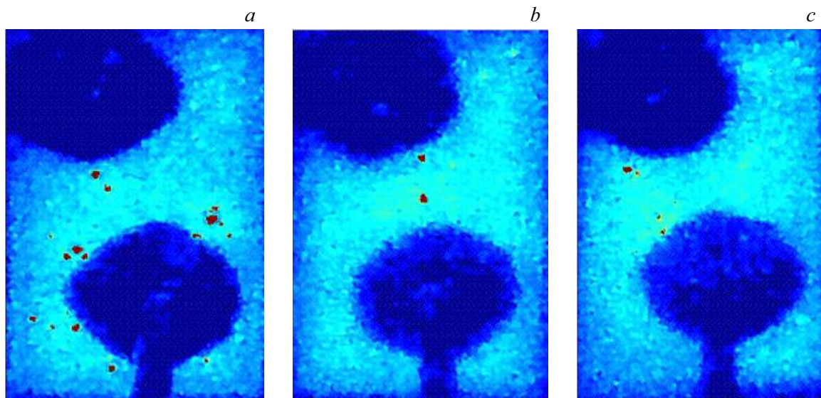
Рис. 4. Изображения кристаллов трех светодиодов в режиме МП пробоя: (а) K = 0.67\% , q = 42830 \text{ A}^{-1} ; (б) K = 0.14\% , q = 48293 \text{ A}^{-1} ; (с) K = 0.10\% , q = 62026 \text{ A}^{-1} .
