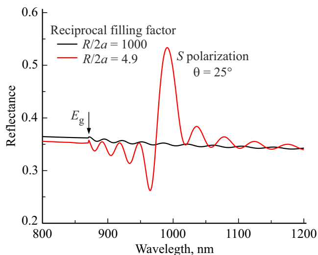
Рис. 3. Результаты моделирования спектров оптического отражения от структуры с 24 эквидистантными квазидвумерными слоями наночастиц Bi с обратным фактором заполнения 4.9 и периодом 139 nm (красная линия) и такой же структуры с обратным фактором заполнения 1000 (черная линия). Расчеты выполнены для S -поляризации и угла падения света 25^\circ .
