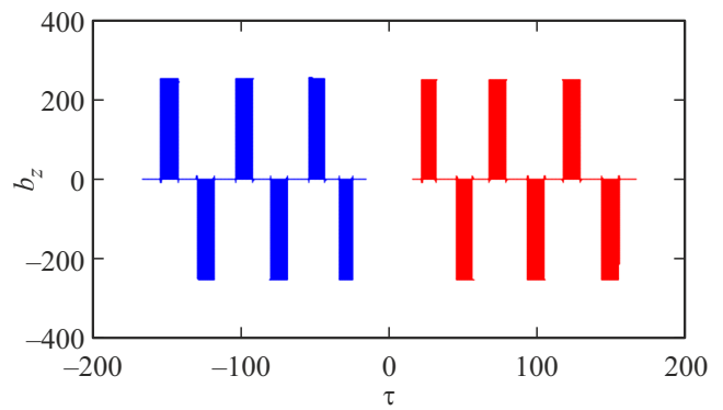
Рис. 4. Безразмерное поле излучения b_z как функция безразмерного времени \tau для нити электронов длиной 2l = \lambda/2 в положительном (красные столбики) и отрицательном направлениях оси Y (синие столбики) в симметричных по y точках пространства (в отсутствие амбиполярного электрического поля).
