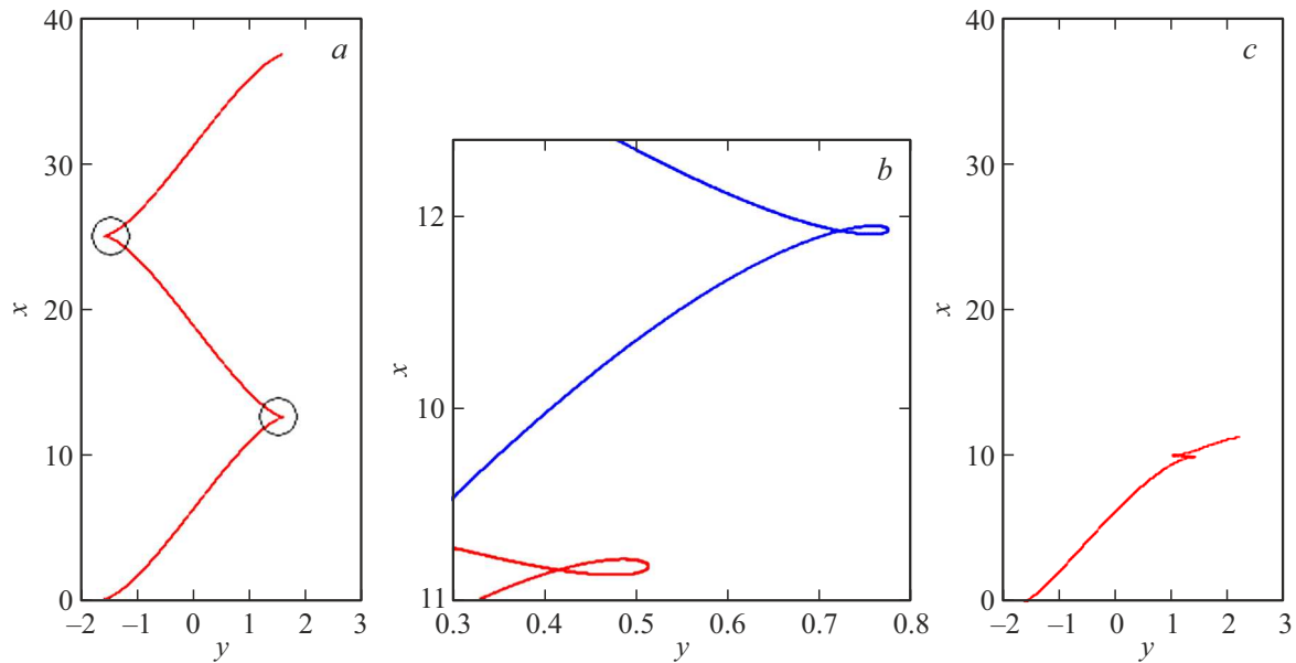
Рис. 1. Траектория с учетом амбиполярных полей: (а) — полей нет; (б) — траектория электрона вблизи вершины (области максимального ускорения) при наличии амбиполярного поля для двух значений тормозящего амбиполярного поля (синяя кривая), \epsilon_x = -1.0 (красная кривая), \epsilon_y = 0 , a_0 = 10 ; (с) траектория электрона при наличии двух компонент амбиполярного поля \epsilon_y = 0.4 , \epsilon_x = -0.4 , a_0 = 10 .
