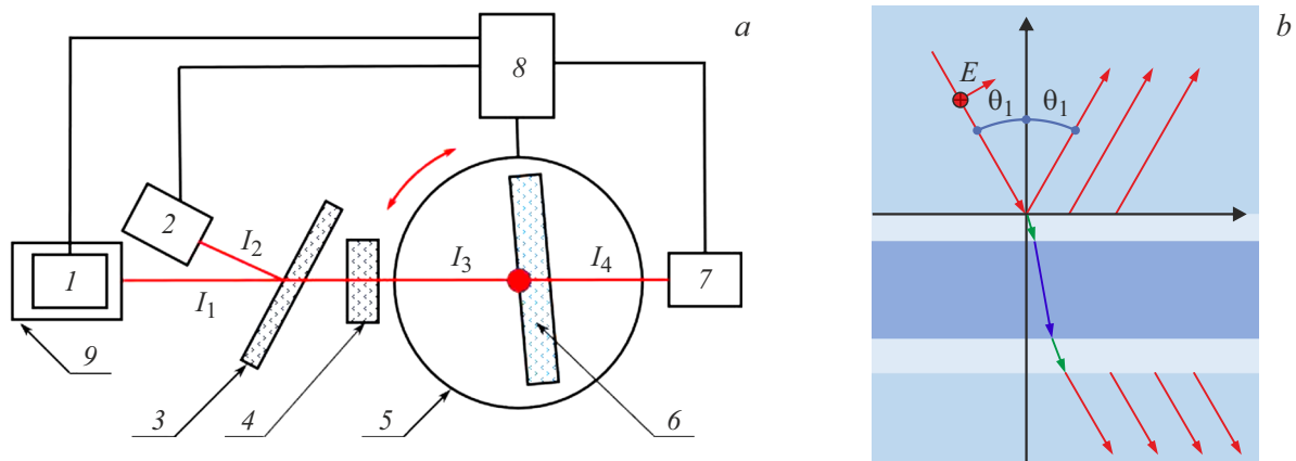
Рис. 1. (а) Схема измерительного стенда. 1 — твердотельный одночастотный лазер BLD-1550-BF-20. 2, 7 ИК фотоприёмники РМ-100. 3 — клиновидный делитель пучка. 4 — призма Глана. 5 — юстировочный узел на базе программно-управляемого поворотного столика Thorlabs HDR50. 6 — образец. 8 — автоматизированный блок управления юстировочным узлом и записи измеряемых параметров. 9 — блок температурной стабилизации лазерного диода; (б) схема, поясняющая расположение слоёв в модели пятислойной симметричной структуры. Прохождение лучей света показано стрелками. Обозначения слоёв сверху вниз: показатели преломления \{n_1 = 1, \tilde{n}_2, n_3, \tilde{n}_2, n_1 = 1\} ; толщины \{d_1 = \infty, d_2, d_3, d_2, d_1 = \infty\} .
