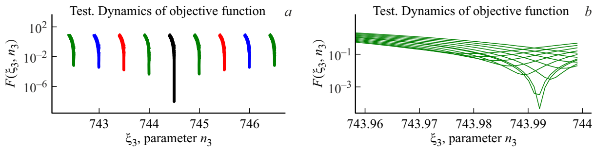
Рис. 3. (а) Динамика целевой функции. Параметр семейства кривых — n_2 (черным цветом обозначен нулевой карман); (b) динамика целевой функции в минус первом кармане.
