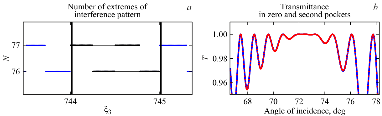
Рис. 4. (а) Число экстремумов интерференционной картины; (b) коэффициент пропускания, при параметрах, определяемых нулевым (синяя линия) и вторым (красный пунктир) карманами (табл. 1).
