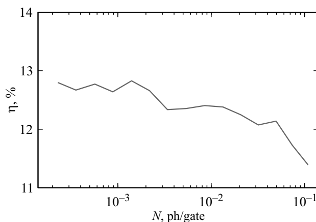
Рис. 2. Измеренная квантовая эффективность детектора SPD-NIR AUREA Technology в зависимости от регистрируемого среднего числа фотонов на строб при следующих параметрах: частота стробирования f_{st} = 1.25 MHz, длительность строба \Delta t = 20 ns, заданная квантовая эффективность \eta = 10\% , мертвое время 0.8 \mu s .
