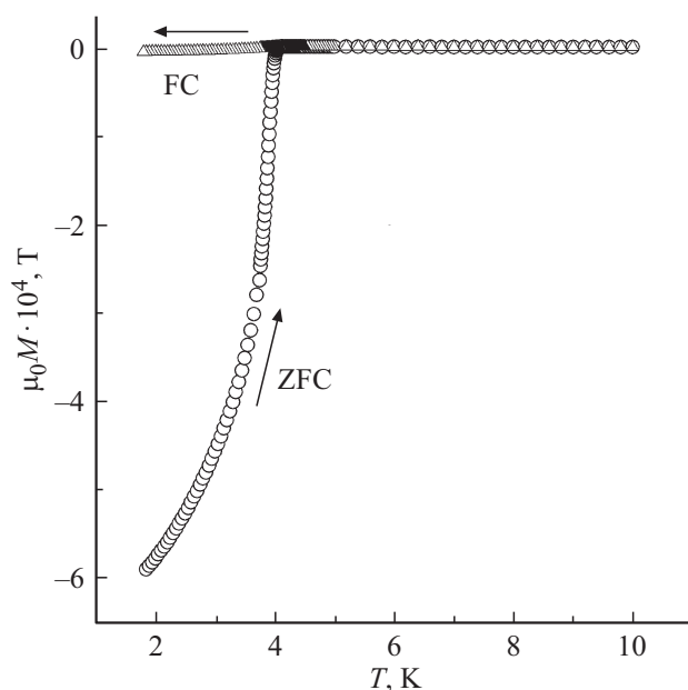
Рис. 1. Температурные зависимости намагниченности, измеренные в режимах ZFC (кружки) и FC (треугольники) во внешнем поле 10 Г. Стрелки показывают направление изменения температуры.
