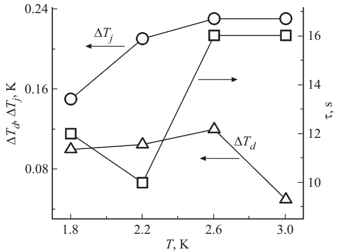
Рис. 5. Температурная зависимость подгоночных параметров \Delta T_j (кружки) и \Delta T_d (треугольники), равных увеличению температуры при скачке намагниченности и времени релаксации \tau , входящего в уравнение (19).
