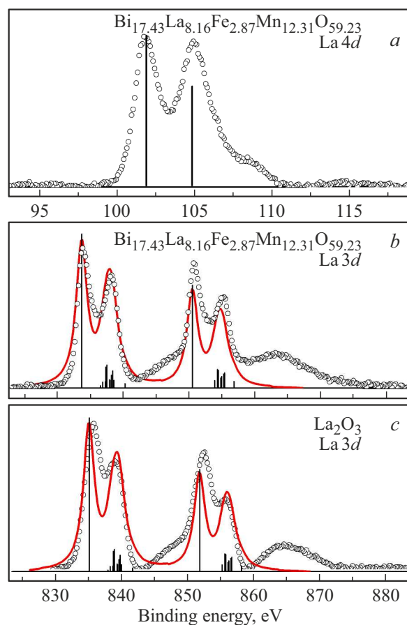
Рис. 4. Спектры La3d -, La4d -уровней для композитного соединения Bi_{17.43}La_{8.16}Fe_{2.87}Mn_{12.31}O_{59.23} и спектр La3d -уровня для соединения La_2O_3 [21]. Кружки — эксперимент, столбики и сплошная линия — расчет.
