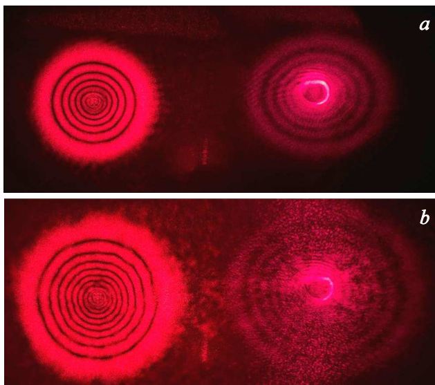
Рис. 2. Дифракция возбуждающего (слева) и зондирующего (справа) пучков для образца с концентрацией магнитной фазы 2 vol.% при H = 0 ( a ) и 700 Ое ( b ).
