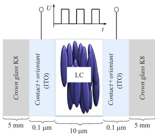
Рис. 1. Структура ЖК-ячейки.
