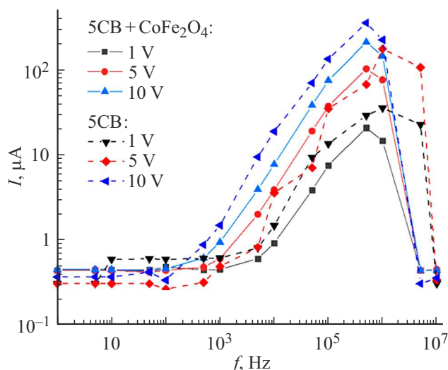
Рис. 2. Зависимость амплитуды силы тока от частоты при различных амплитудах прикладываемого синусоидального напряжения.
