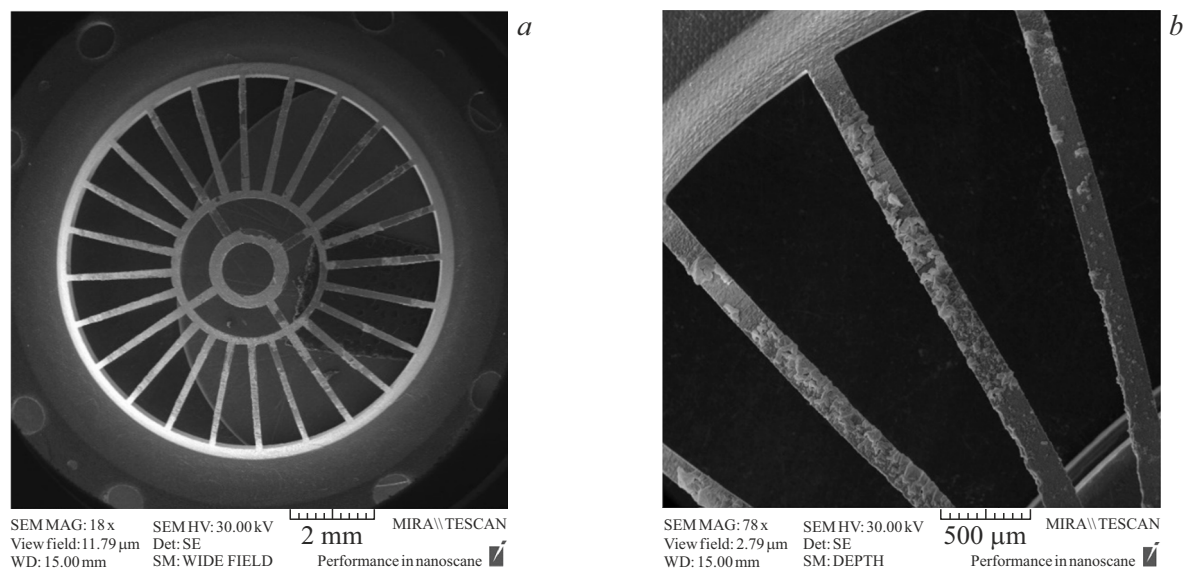
Рис. 3. Управляющая сетка. Вид со стороны катода: a — общий вид, b — периферийная часть.
