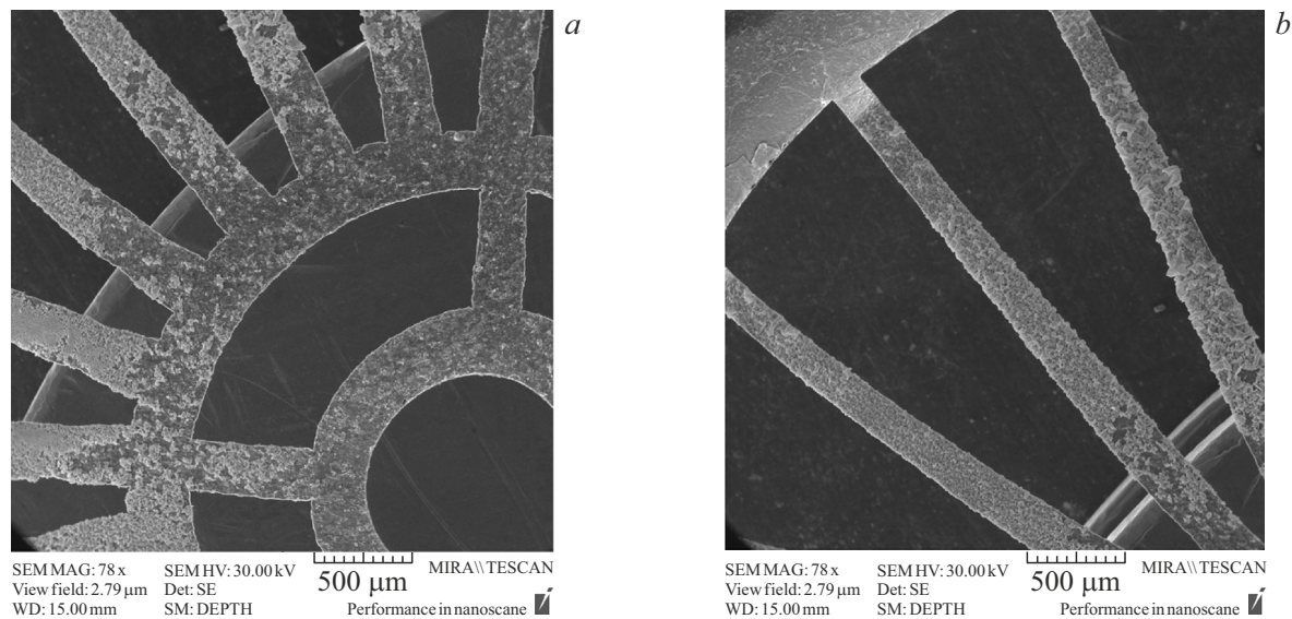
Рис. 2. Теневая сетка. Вид со стороны катода: a — центральная часть с кольцевыми перемычками, b — периферийная часть с радиальными перемычками.
