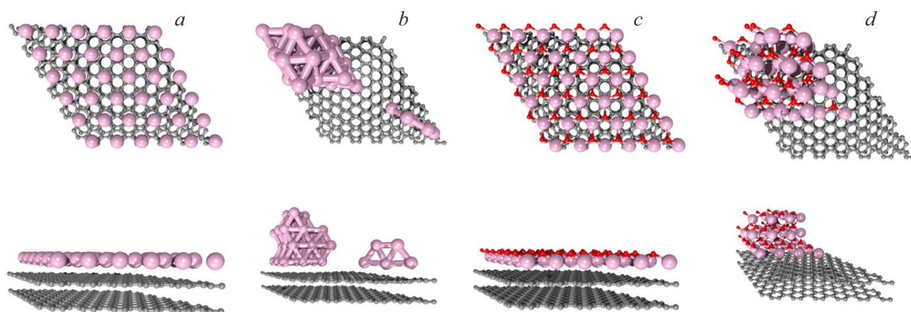
Рис. 4. Суперъчейки атомистических моделей пленок „АПГ + Ba/BaO“: a — однородное распределение бария; b — неоднородное распределение бария; c — однородное распределение BaO; d — неоднородное распределение BaO (серым цветом отмечены атомы углерода, розовым — бария, красным — кислорода). Здесь АПГ представлен двумя углеродными слоями.
