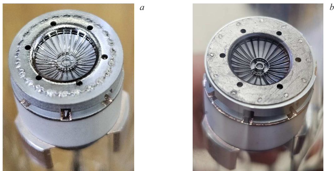
Рис. 1. Общий вид КСУ с сетками ажурной конструкции из гафния (а) и из АПГ (b).
