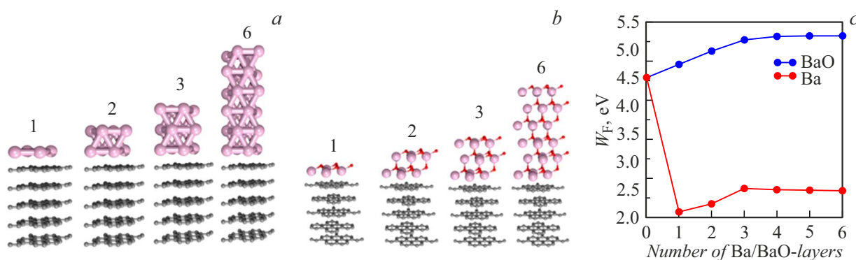
Рис. 5. Пленки „АПГ + Ba/BaO“: a — атомистические ячейки моделей пленок „АПГ + Ba“; b — атомистические ячейки моделей пленок „АПГ + BaO“; c — график изменения работы выхода при наращивании количества слоев Ba/BaO.
