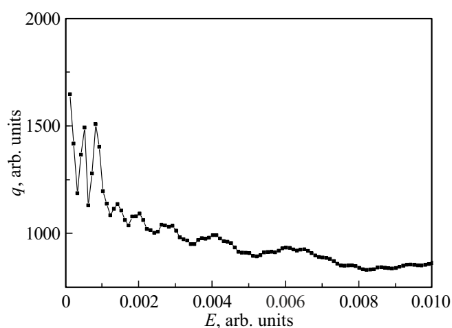
Рис. 4. Зависимость полного сечения упругого рассеяния ( q_{\text{tot}} ) от энергии столкновения для пары ^{23}\text{Na}-^{85}\text{Rb} в атомной системе единиц.
