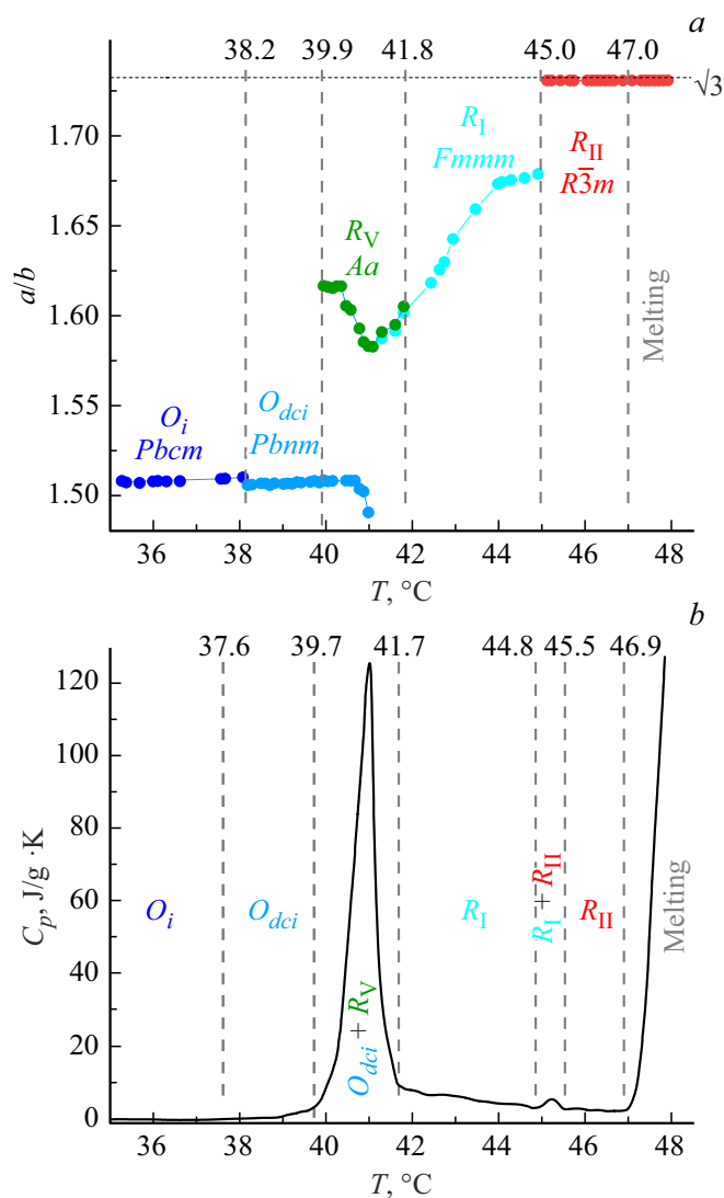
Рис. 8. a — температурные изменения отношения параметров элементарных ячеек a/b полиморфных модификаций трикозана при нагревании в температурном интервале \Delta T = 35.0\text{--}48.0^\circ\text{C} ; b — полиморфные модификации трикозана на ДСК термограмме.
