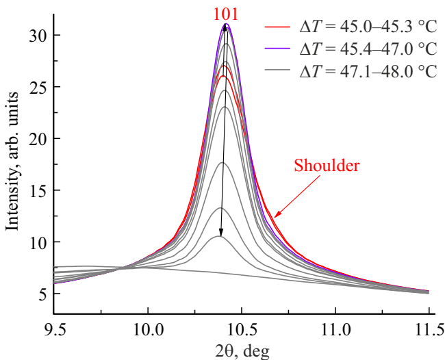
Рис. 6. Температурные изменения дифрактограмм трикозана при нагревании в температурном интервале \Delta T = 45.0\text{--}48.0^\circ\text{C} . Черными стрелками указаны направления изменений при нагревании. Красная стрелка подчеркивает наличие плеча у рефлекса 101, обусловленного остатками орторомбической фазы. Красным цветом представлены дифрактограммы сосуществования фаз R_I и R_{II} , фиолетовым — фазы R_{II} , серым — плавления образца.
