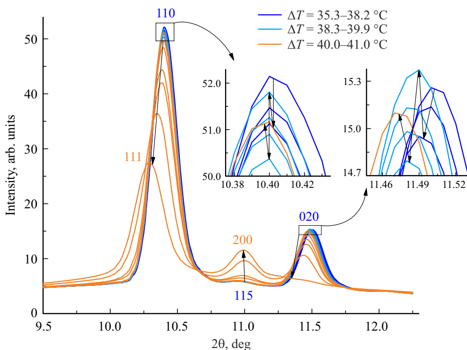
Рис. 3. Температурные изменения дифрактограмм трикозана при нагревании в температурном интервале \Delta T = 35.3\text{--}41.0\text{ }^{\circ}\text{C} . На вставках представлены более детально изменения рефлексов. Стрелками указаны направления изменений при нагревании. Синим цветом представлены дифрактограммы фазы O_i , голубым — фазы O_{dci} , оранжевым — сосуществования фаз O_{dci} и R_V .
