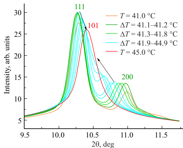
Рис. 5. Температурные изменения дифрактограмм трикозана при нагревании в температурном интервале \Delta T = 41.0\text{--}45.0^\circ\text{C} . Стрелками указаны направления изменений при нагревании. Оранжевым цветом представлены дифрактограммы сосуществования фаз O_{dci} и R_V , зеленым — фазы R_V , светло зеленым — промежуточного состояния между R_V и R_I , бирюзовым — фазы R_I , красным — сосуществования фаз R_I и R_{II} .
