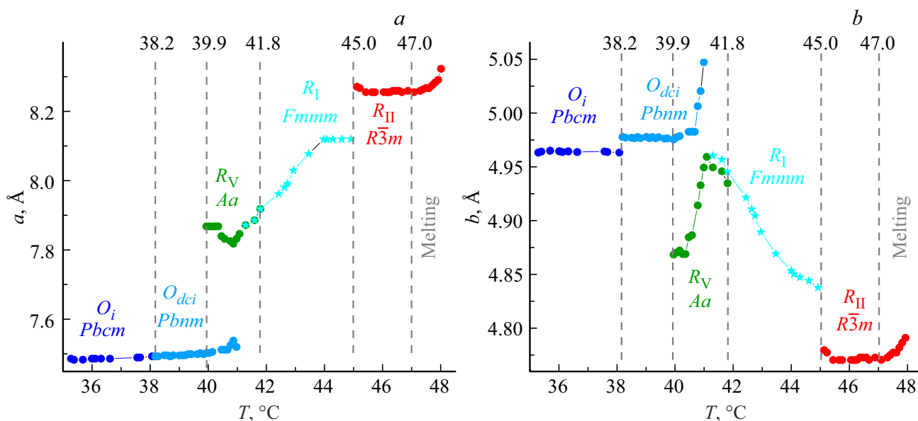
Рис. 7. Температурные изменения параметров a (а) и b (б) элементарных ячеек полиморфных модификаций трикозана при нагревании в температурном интервале \Delta T = 35.0\text{--}48.0^\circ\text{C} .
