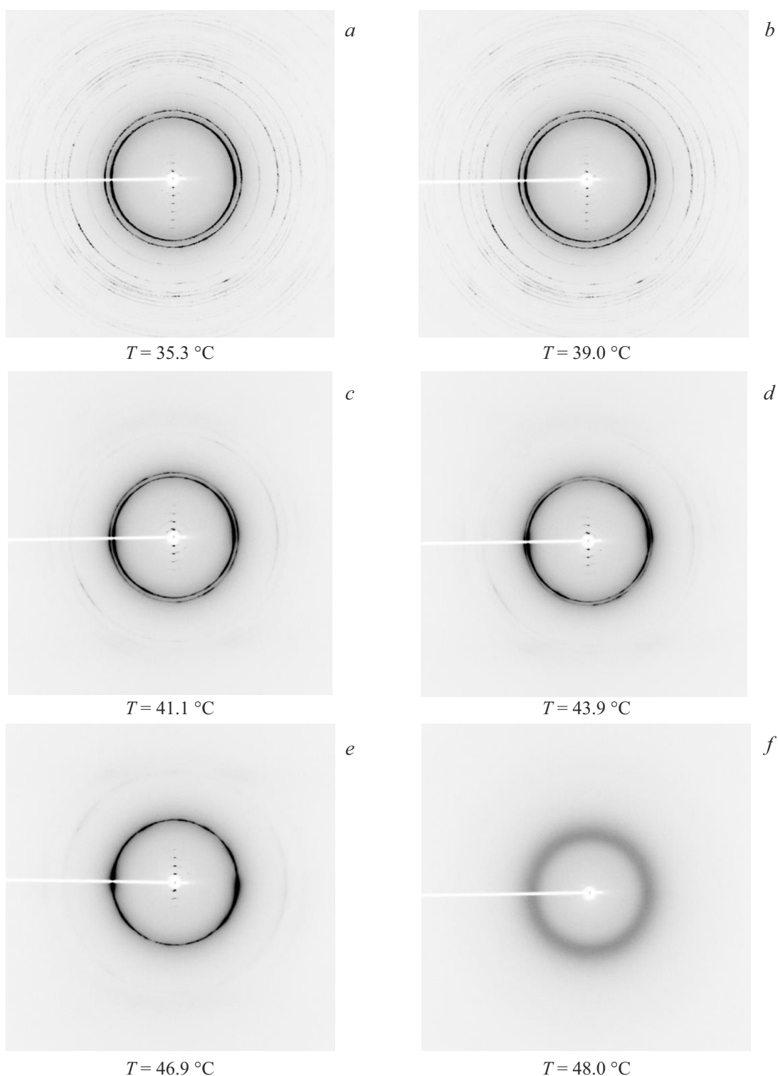
Рис. 2. 2D-дифрактограммы триолеина, каждая из которых получена в интервале нагрева \Delta T = 0.06\text{ }^{\circ}\text{C} и обозначена средней температурой: 35.3 (a), 39.0 (b), 41.1 (c), 43.9 (d), 46.9 (e), 48.0 ^{\circ}\text{C} (f).
