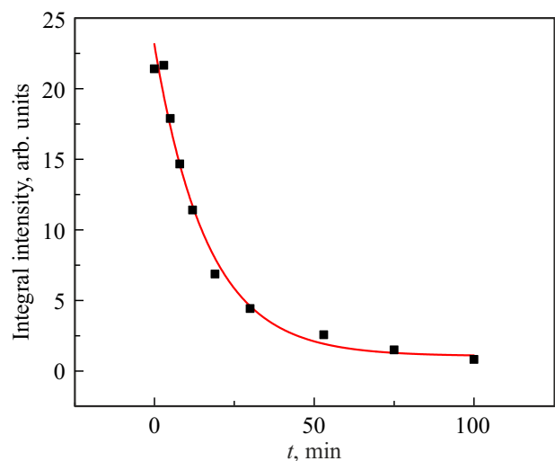
Рис. 4. Зависимость интегральной интенсивности полосы поглощения 490 nm УТ от времени УФ облучения t . Точки — экспериментальные данные, сплошная линия — аппроксимация экспериментальной зависимости уравнением (4).
