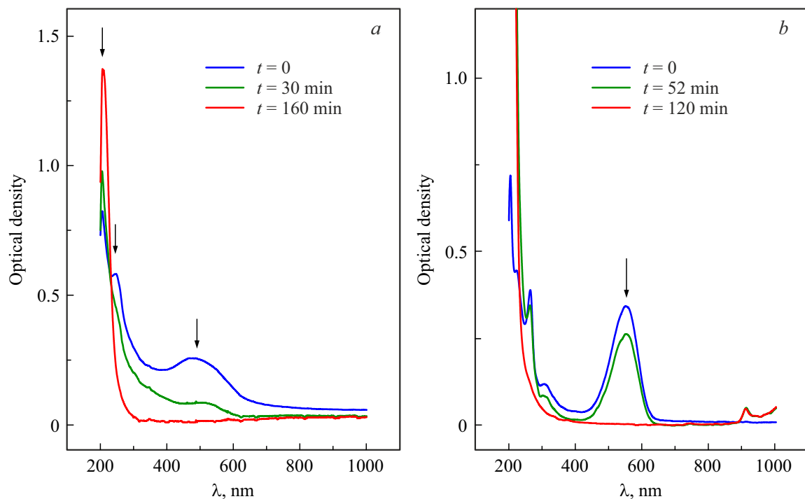
Рис. 3. Влияние УФ облучения на спектры поглощения УТ (а) и НК (b) в этаноле. Время облучения t указано на вставке.
