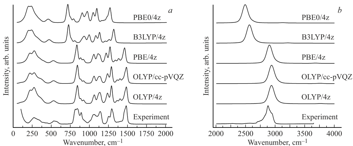
Рис. 2. Экспериментальный спектр КР образца ПЭГ400, измеренный при длине волны возбуждающего излучения 785 nm, рассчитанные и уширенные спектры КР нонамера ЭГ в приближениях OLYP/4z, OLYP/cc-pVQZ, PBE/4z, B3LYP/4z и PBE0/4z: диапазоны 100–2000 (a), 2000–4000 \text{cm}^{-1} (b).
