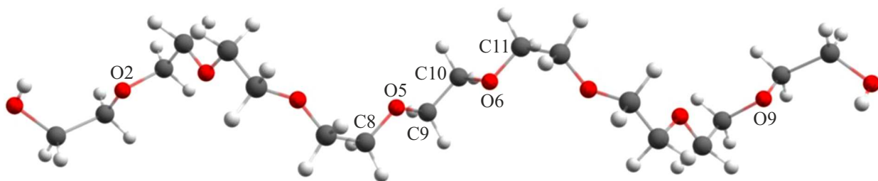
Рис. 3. Структура нонамера ЭГ, оптимизированная в приближении OLYP/4z. Серым цветом показаны атомы углерода, белым цветом — атомы водорода, красным цветом — атомы кислорода.
