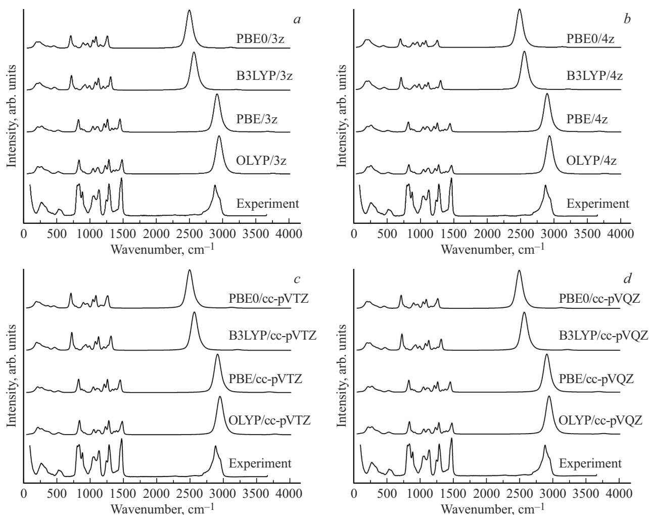
Рис. 1. Экспериментальный спектр КР образца ПЭГ400, измеренный при длине волны возбуждающего излучения 785 nm, рассчитанные и уширенные спектры КР нонамера ЭГ, полученные с использованием функционалов электронной плотности OLYP, PBE, B3LYP и PBE0 и следующих базисных наборов: 3z (a), 4z (b), cc-pVTZ (c), cc-pVQZ (d).
