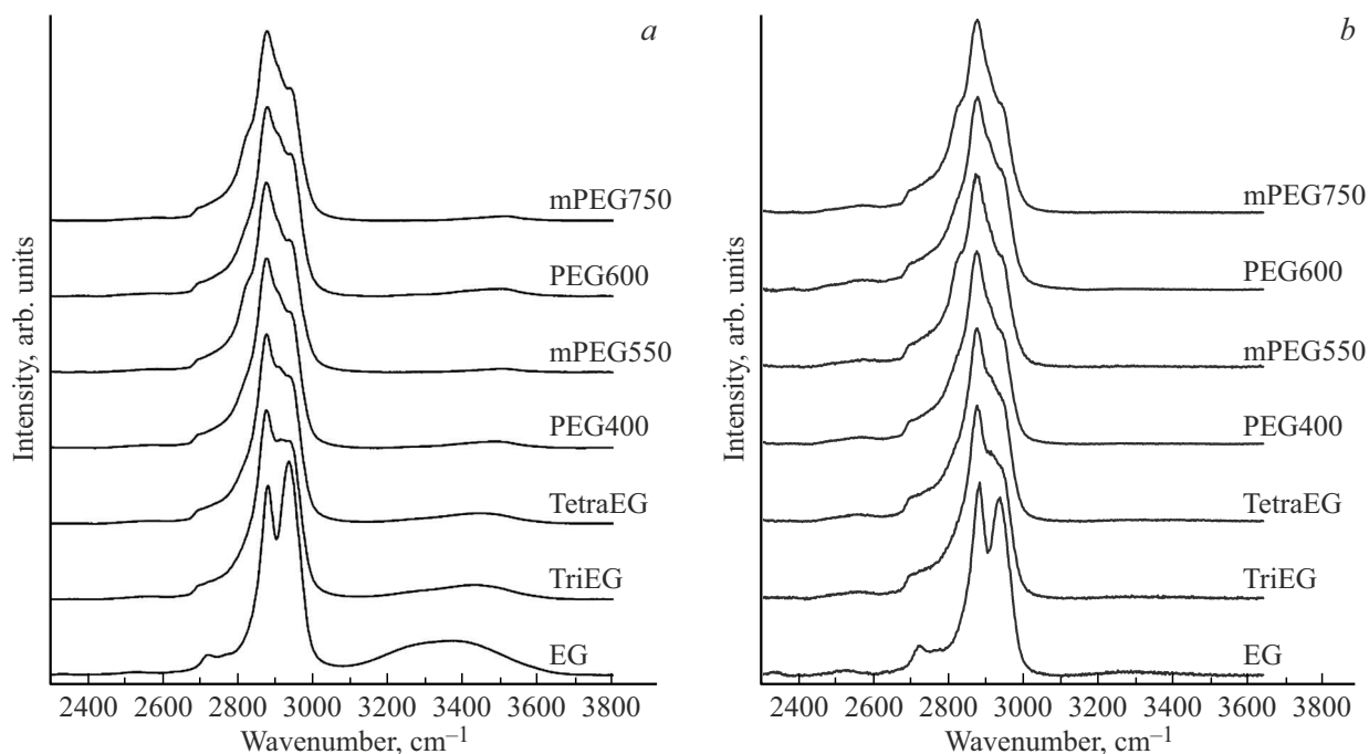
Рис. 5. Спектры КР ЭГ, ПЭГ и мПЭГ, записанные при длине волны возбуждения 532 (a) и 785 nm (b), диапазон II.
