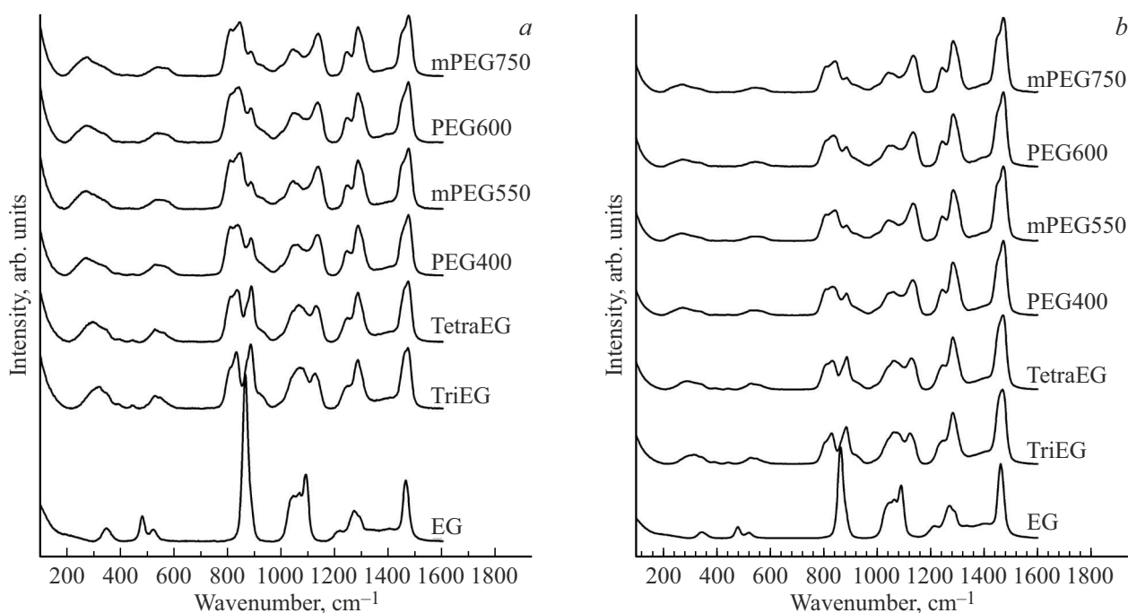
Рис. 4. Спектры КР ЭГ, ПЭГ и мПЭГ, записанные при длине волны возбуждения 785 (a) и 532 nm (b), диапазон I.
