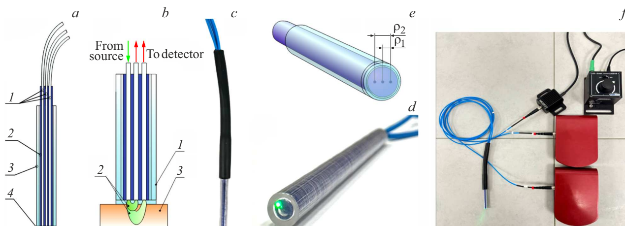
Рис. 1. Сапфировый зонд для определения оптических свойств тканей в условиях нарушенной микроциркуляции. (а) Схема сапфирового зонда: 1 — оптические волокна, 2 — пластиковая трубка, 3 — сапфировая трубка, 4 — сапфировая пластинка. (б) Оптическая схема: 1 — зонд, 2 — ход лучей, 3 — биологическая ткань. (с), (д) Фотографии сапфирового зонда. (е) Вид контактной части зонда, \rho_1 = 1.3 и \rho_2 = 2.6 mm. (ф) Фотография экспериментальной установки.
