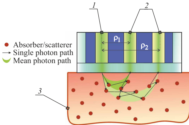
Рис. 3. Ход лучей в образце ткани, регистрируемых каналами детектора: 1 — излучательное волокно, 2 — детектирующие волокна, 3 — образец ткани.
