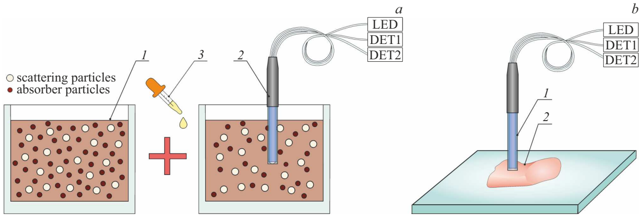
Рис. 2. Иллюстрация экспериментов с фантомами ткани и образцами мышечной ткани. (а) Измерение параметров фантома, состоящего из липидной эмульсии с добавлением гемоглобина до и после добавления сычужного фермента: 1 — фантом, 2 — сапфировый зонд, 3 — сычужный фермент. (б) Измерение параметров образца мышечной ткани: 1 — сапфировый зонд, 2 — образец ткани.
