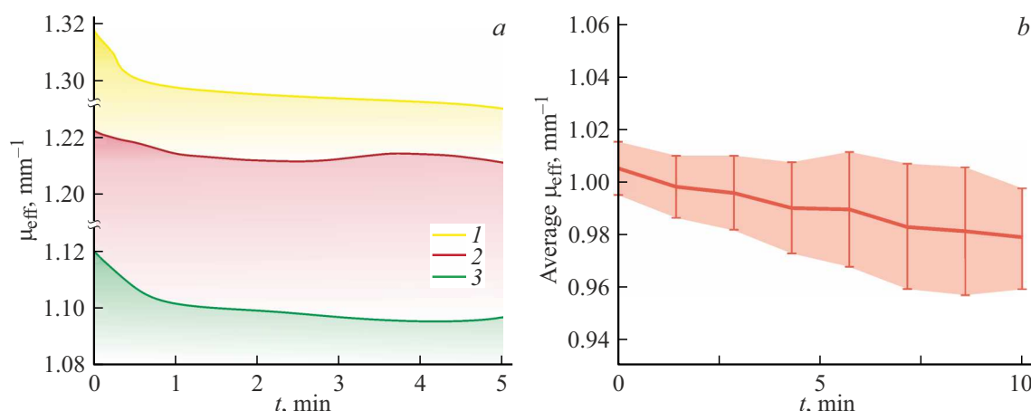
Рис. 4. Измерение эффективного коэффициента ослабления образцов с помощью сапфирового зонда. (а) Изменение во времени эффективного коэффициента ослабления фантома ткани после добавления сычужного фермента: 1 — для 0.05 g гемоглобина, 2 — для 0.10 g гемоглобина, 3 — для 0.15 g гемоглобина. (б) Среднее значение эффективного коэффициента ослабления образцов мышечной ткани.
