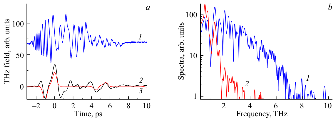
Рис. 2. (a) — временные профили ТГц импульсов, полученные для случая лазерного излучения длительностью 30 fs (1), 250 fs (2), моделирование для случая 250 fs (3); (b) — соответствующие спектры ТГц импульсов (1) и (2).
