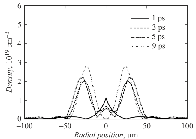
Рис. 1. Динамика поперечного распределения плотности плазмы аргона в канале, создаваемом лазерным импульсом с энергией 90 мДж, длительностью импульса 0.3 нс, длина волны лазера 0.8 мкм [22].
