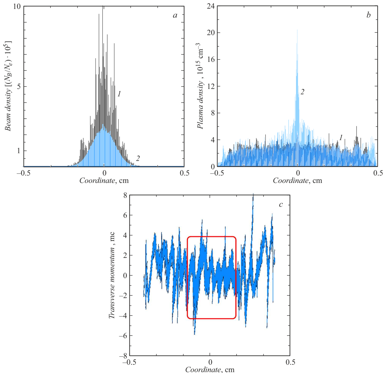
Рис. 3. Параметры пучка протонов с зарядом 50 pC и энергией 250 MeV после прохождения расстояния 10 см в однородной плазме с плотностью N_e = 10^{15} \text{ cm}^{-3} в момент времени t = 0 ; a — профиль протонного пучка после прохождения плазмы (1) и на входе в плазму (2); b — профиль электронов и ионов плазмы, формируемой лазерным импульсом с ponderomotorным потенциалом \sim 9 \text{ keV} ; c — распределение поперечного импульса протонов в пучке после прохождения плазмы, выделенная область показывает расположение пучка протонов в пределах сигмы, т.е. в области максимальной плотности пучка.
