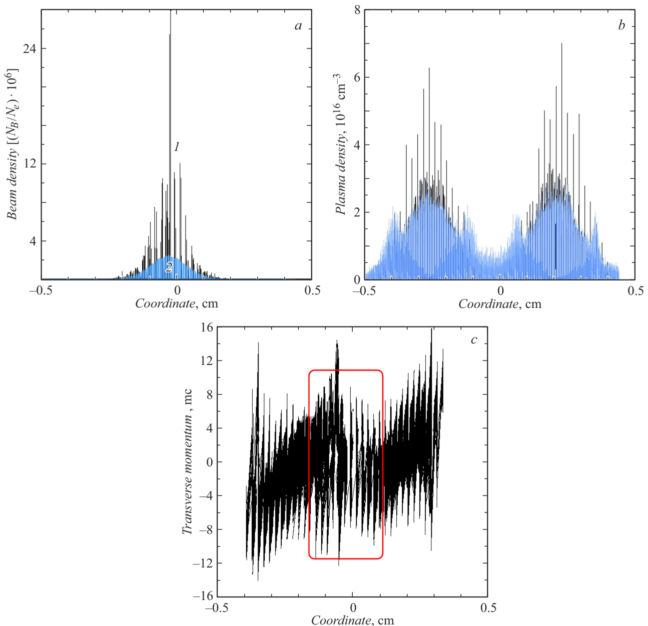
Рис. 4. Параметры пучка протонов с зарядом 50 pC и энергией 250 MeV после прохождения расстояния 10 см в плазме с плотностью N_e = 10^{15} \text{ cm}^{-3} , формируемой радиально поляризованным лазерным импульсом; a — профиль протонного пучка после прохождения плазмы (1) и на входе в плазму (2); b — профиль электронов и ионов плазмы, формируемой поперечным потенциалом 9 keV; c — распределение поперечного импульса протонов в пучке после прохождения плазмы, выделенная область показывает расположение пучка протонов в пределах сигмы.
