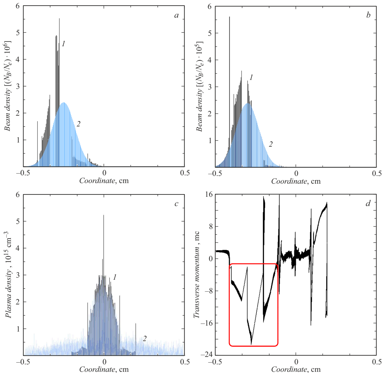
Рис. 5. Параметры пучка протонов с зарядом 50 pC и энергией 250 MeV после прохождения расстояния 10 cm в плазме с плотностью N_e = 10^{15} \text{ cm}^{-3} с поперечным размером сравнимым с поперечным размером пучка; a, b — профили протонного пучка, смещенного относительно центра плазмы на 2, 5 и 3 mm, после прохождения плазмы (1) и на входе в плазму (2); c — профиль электронов и ионов плазмы, формируемой пондеромоторным потенциалом 9 keV; d — распределение поперечного импульса протонов в пучке после прохождения плазмы с параметрами как на рис. 5, b , выделенная область показывает расположение пучка протонов в пределах сигмы, т. е. в области основной плотности пучка.
