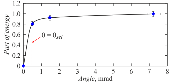
Рис. 9. Угловое распределение энергии излучения лазера с сопряженным резонатором, содержащим ПВМС с двойным поворотом плоскости поляризации на 90^\circ .
