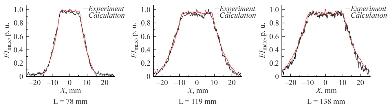
Рис. 4. Профили распределения интенсивности, зарегистрированные в эксперименте и рассчитанные в программном пакете.
