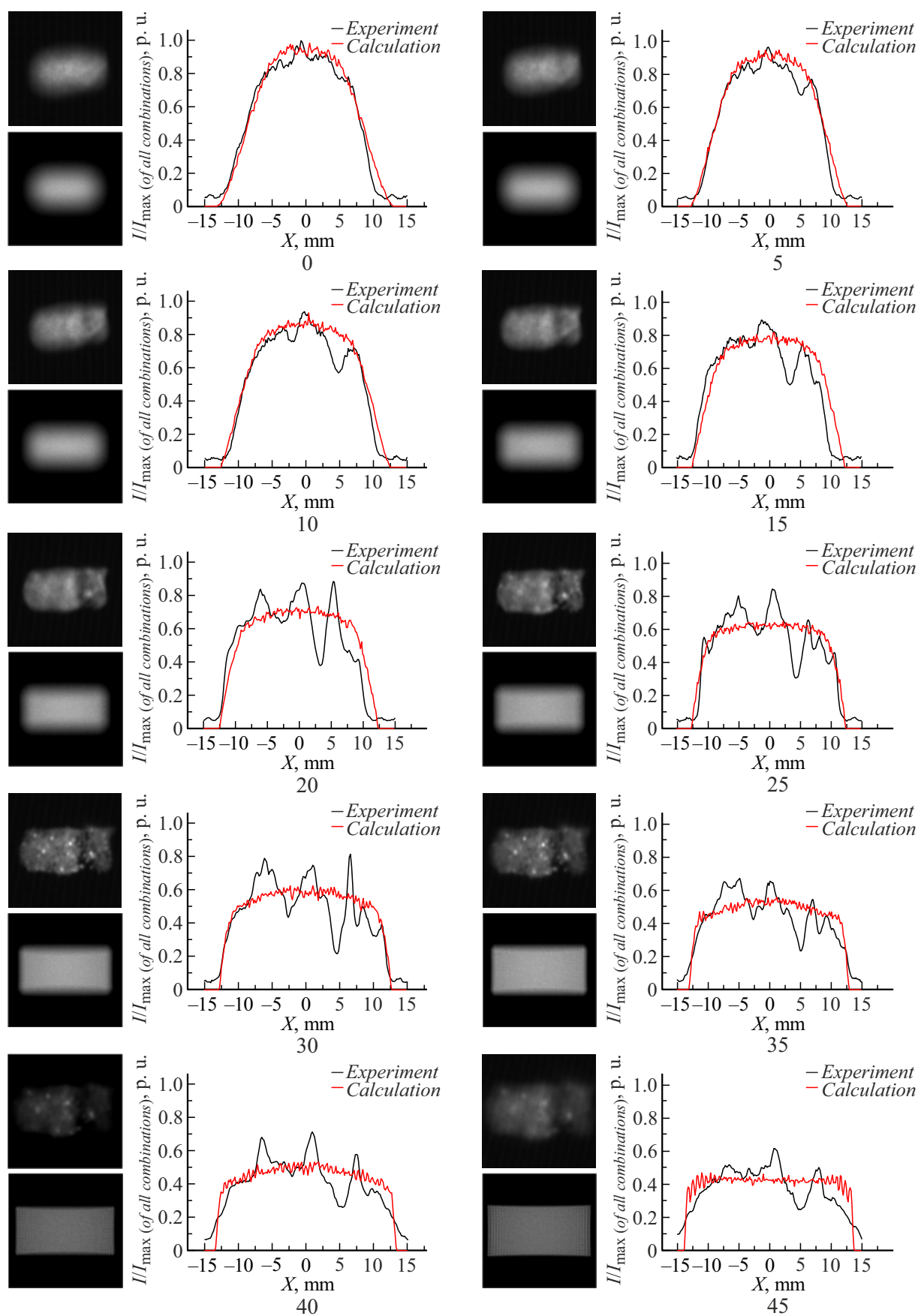
Рис. 7. Экспериментальные и расчетные распределения интенсивности внутри лазерной кюветы от тела свечения 20.5 \times 10.5 mm.
