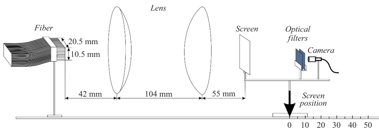
Рис. 5. Схема регистрации распределения интенсивности излучения накачки внутри кюветы от тела свечения 20.5 \times 10.5 mm.
