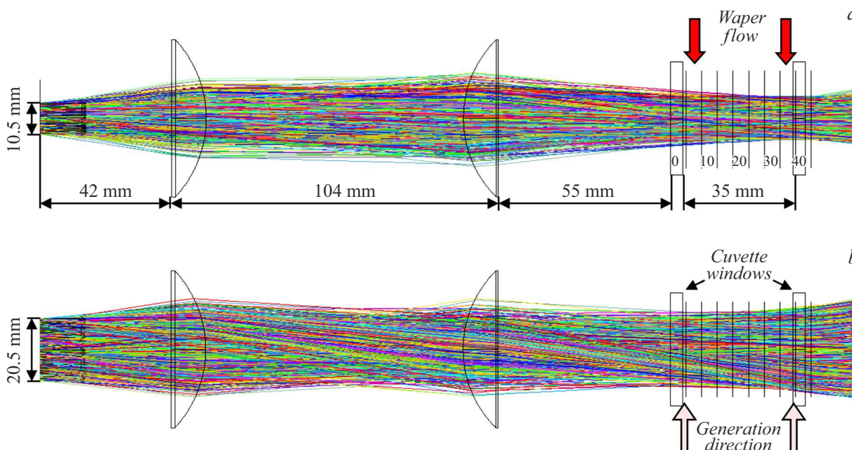
Рис. 6. Оптическая схема системы ввода излучения накачки в лазерную кювету: a — вид сбоку (по направлению генерации), b — вид сверху (по направлению потока паров рубидия).
