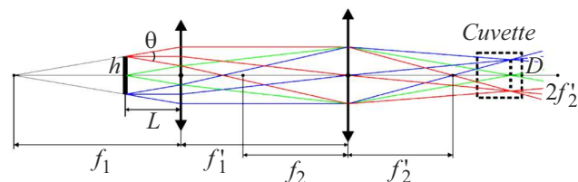
Рис. 1. Перестроение изображения источника излучения в кювету лазера: h — размер источника, \theta — расходимость излучения, L — расстояние от источника до линзы, D — поперечный размер области накачки, f_1' , f_1 ; f_2' , f_2 — фокусные расстояния первой и второй линз.
