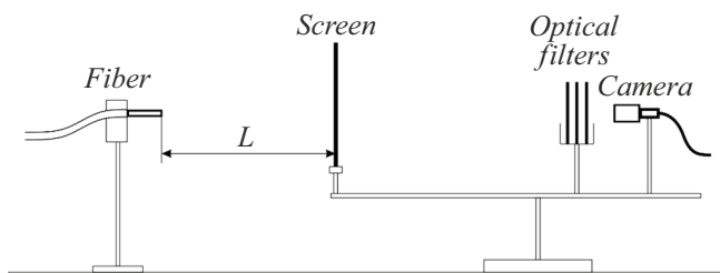
Рис. 2. Схема эксперимента.
