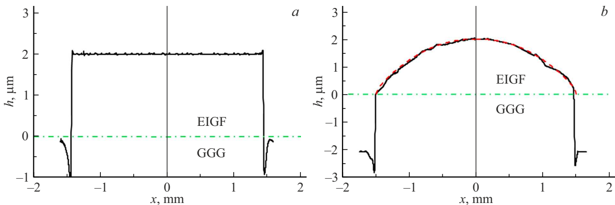
Рис. 10. Профиль поперечного сечения сформированной поверхности с использованием маски в виде диска ( a ) и последующим наложением сферической маски ( b ). Штрихпунктиром отмечена граница между пленкой ЭПФГ и подложкой ГГГ, пунктиром показана модельная аппроксимация гладкого профиля травления.
