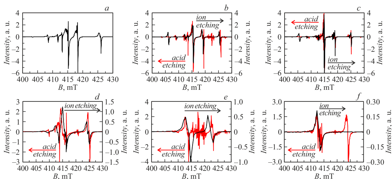
Рис. 5. Резонансные кривые ФМР (пленка (\text{YLa})_3(\text{FeGaAl})_5\text{O}_{12} , h = 2.1 \mu\text{m} ) для перпендикулярного ( 0^\circ ) резонанса (красная линия — кислотное травление, черная линия — ионное травление); a — квадрат ( h = 2.1 \mu\text{m} , до обработки), b — диск R = 1.5 mm, c — диск R = 1 mm, d — квадрат ( h = 1.6 \mu\text{m} ), e — квадрат ( h = 1.1 \mu\text{m} ), f — квадрат ( h = 0.6 \mu\text{m} ).
