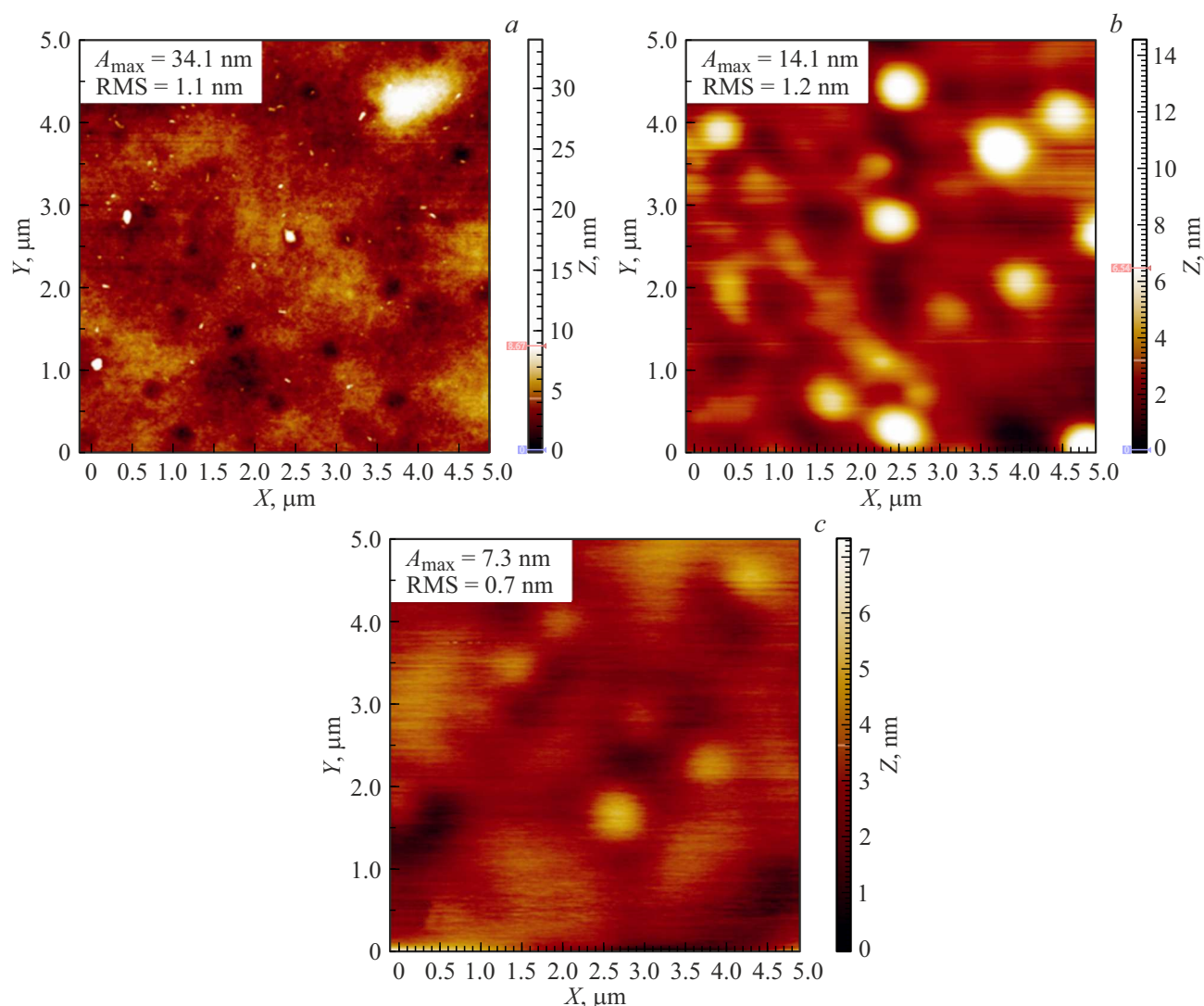
Рис. 3. АСМ анализ морфологии поверхности ЭПФГ (\text{YLa})_3(\text{FeGaAl})_5\text{O}_{12} ( h = 2.1 \mu\text{m} ) после кислотной обработки при травлении слоя толщиной 0.5 (а), 1 (б) и 1.5 \mu\text{m} (с).
