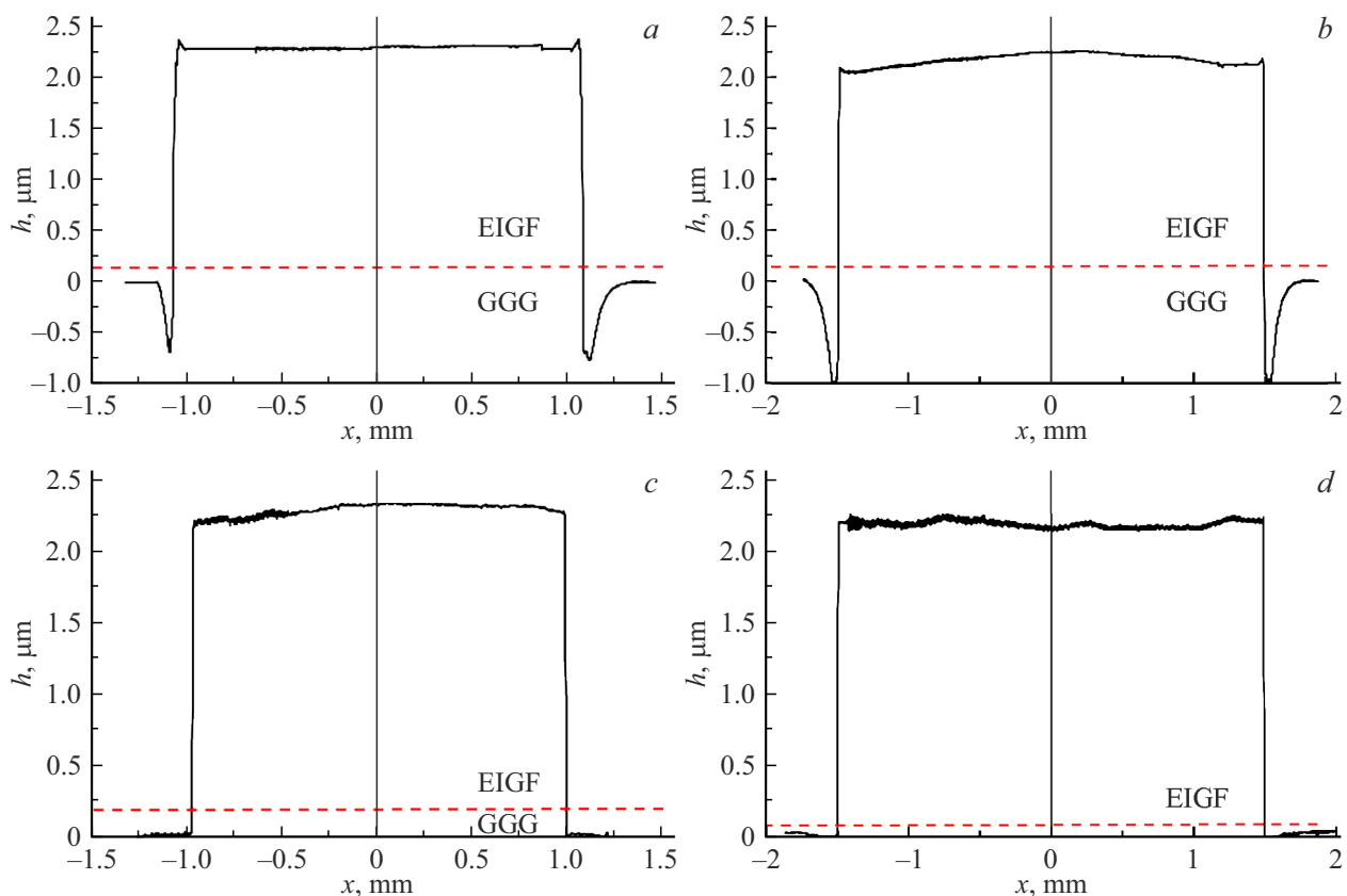
Рис. 1. Профиль поперечного сечения дисков, полученных методами ионно-плазменного травления ( a, b ) и кислотного травления ( c, d ), диски диаметром 2 mm ( a, c ) и диаметром 3 mm ( b, d ). Штриховой линией показана граница между пленкой ЭПФГ и подложкой ГГГ.
