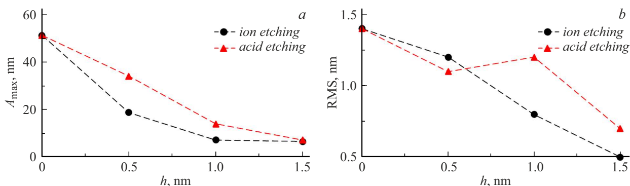
Рис. 4. Изменение параметров шероховатости поверхности ЭПФГ при послойном травлении различными методами; a — параметр A_{\max} , b — параметр RMS.
