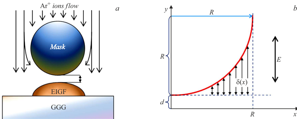
Рис. 8. Ионно-плазменное травление с использованием сферической маски: схема травления (а), рассмотренная модель (b).
