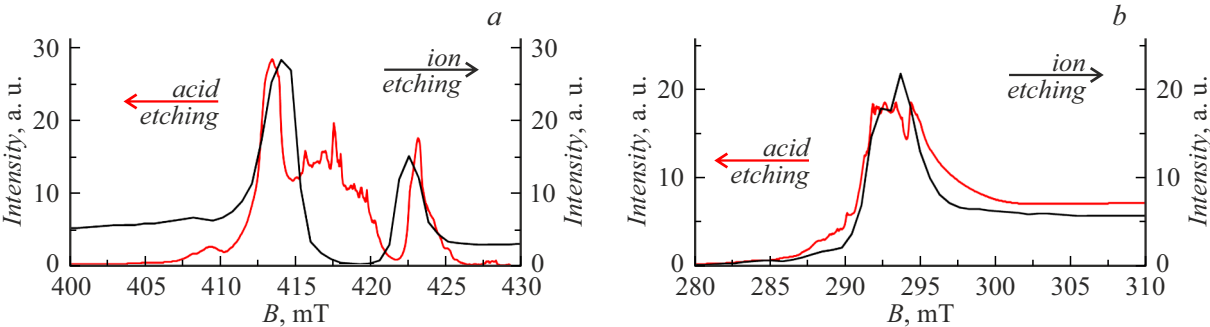
Рис. 7. Пример построения интегральных ФМР спектров на основании дифференциальных (рис. 5, 6) для пленки ЭПФГ толщиной h = 1.1 \mu\text{m} ; a — перпендикулярный резонанс ( 0^\circ ), b — параллельный резонанс ( 90^\circ ).
