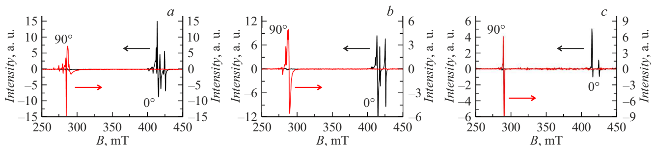
Рис. 11. Резонансные кривые ФМР (пленка (\text{YLa})_3(\text{FeGaAl})_5\text{O}_{12} , h = 2 \mu\text{m} ) для параллельного ( 90^\circ ) и перпендикулярного ( 0^\circ ) резонанса: a — ЭПФГ до обработки; b — диск диаметром 3 mm (рис. 9, a ); c — эллипс диаметром 3 mm (рис. 9, b ).
