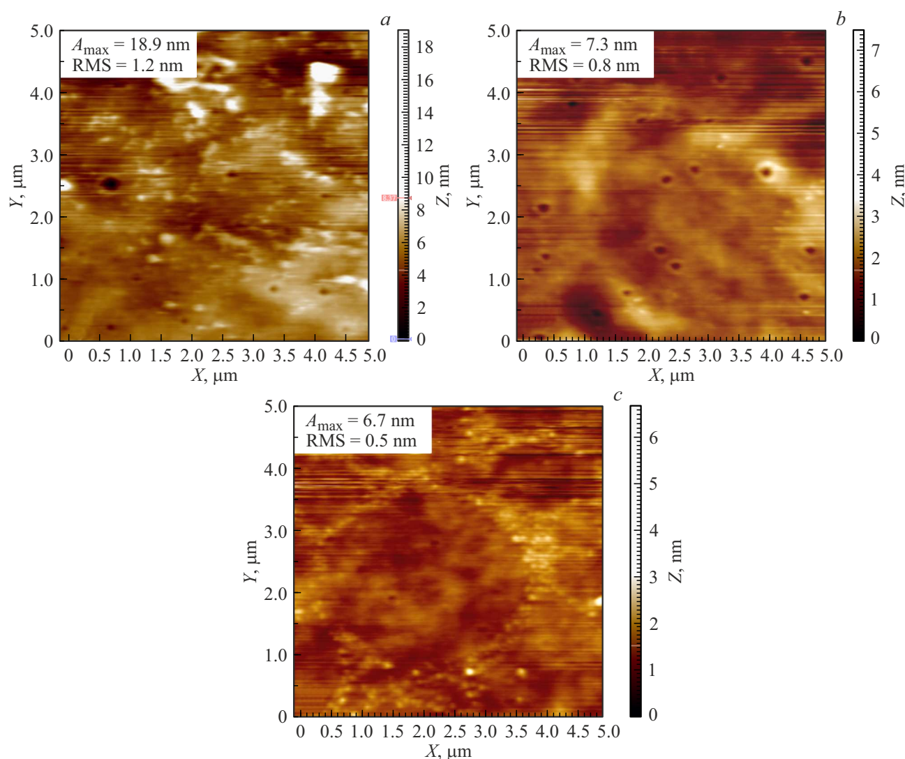
Рис. 2. АСМ анализ морфологии поверхности ЭПФГ (\text{YLa})_3(\text{FeGaAl})_5\text{O}_{12} ( h = 2.1 \mu\text{m} ) после ионной обработки при травлении слоя толщиной 0.5 (a), 1 (b) и 1.5 \mu\text{m} (c).
