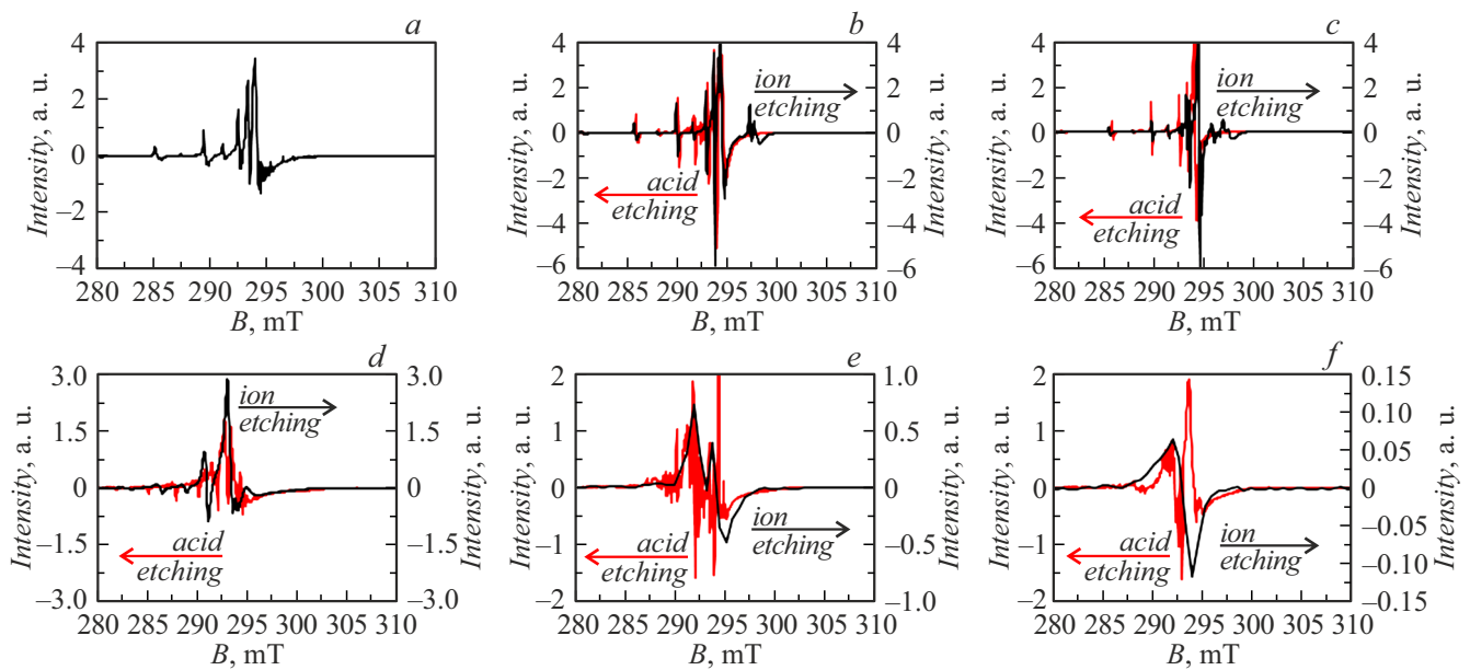
Рис. 6. Резонансные кривые ФМР (пленка (YLa)_3(FeGaAl)_5O_{12} , h = 2.1 \mu m ) для параллельного ( 90^\circ ) резонанса (красная линия — кислотное травление, черная линия — ионное травление); a — квадрат, ( h = 2.1 \mu m , до обработки), b — диск R = 1.5 mm , c — диск R = 1 mm , d — квадрат ( h = 1.6 \mu m ), e — квадрат ( h = 1.1 \mu m ), f — квадрат ( h = 0.6 \mu m ).
