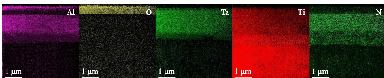
Рис. 10. Карты распределения химических элементов на поперечном сечении покрытия, полученного в режиме МРПТ, на подложке из сплава ВТ6 после отжига при температуре 950 °C в течение 5 h.
