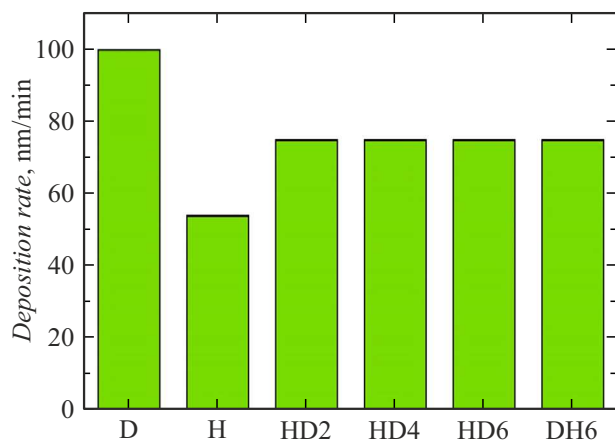
Рис. 1. Скорость осаждения покрытий Ti–Al–Ta–N, полученных в различных режимах.
