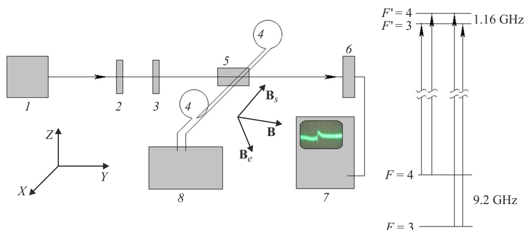
Рис. 1. Схема экспериментальной установки. 1 — перестраиваемый лазер, 2 — аттенюатор, 3 — полуволновая пластинка, используемая для поворота азимута линейной поляризации зондирующего пучка, 4 — соленоид, 5 — кювета с парами Cs, 6 — фотоприемник, 7 — осциллограф, 8 — генератор синусоидального тока. В левом нижнем углу показана лабораторная система координат. Справа приведена схема переходов линии D1 цезия. \mathbf{B}_s — поле соленоида, \mathbf{B}_e — земное поле, \mathbf{B} — полное поле.
