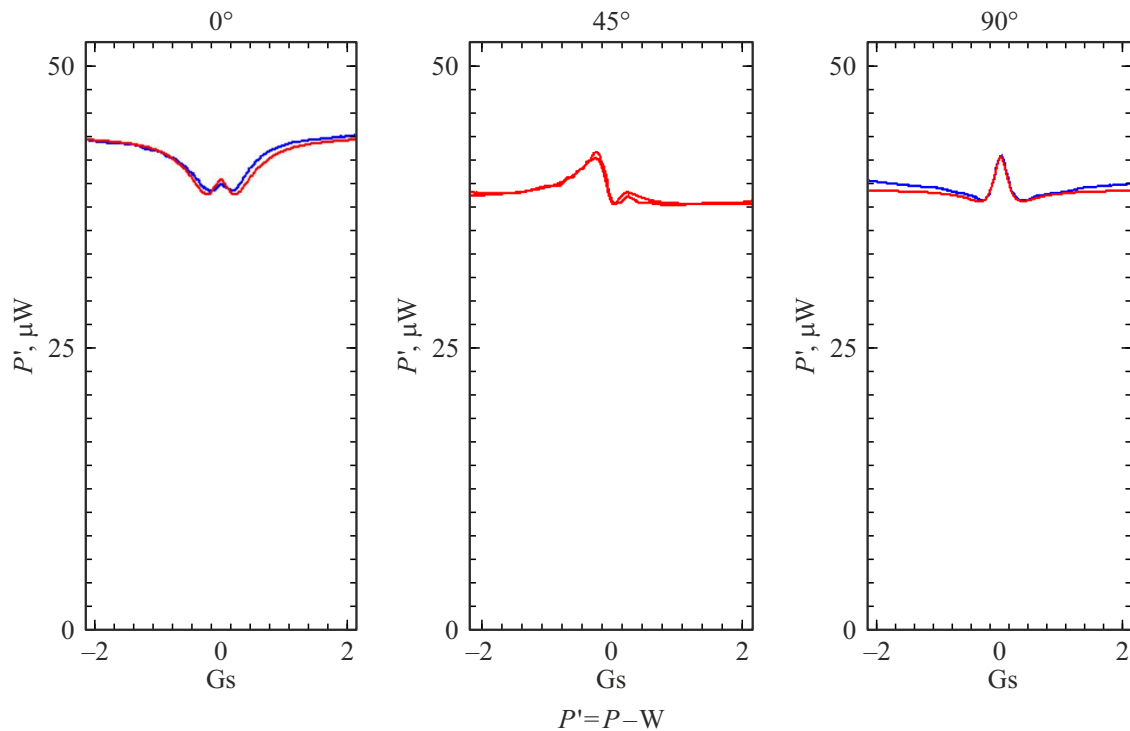
Рис. 5. Резонансное зондирование на переходе F = 4 \rightarrow F' = 3 линии D1 цезия. Расчетные (гладкие) и экспериментальные (зашумленные) зависимости мощности P' пучка, прошедшего через кювету, от магнитного поля соленоида в геометрии Фойхта при различных взаимных ориентациях азимута поляризации зондирующего пучка и магнитного поля соленоида (сравните с рис. 2, c).
