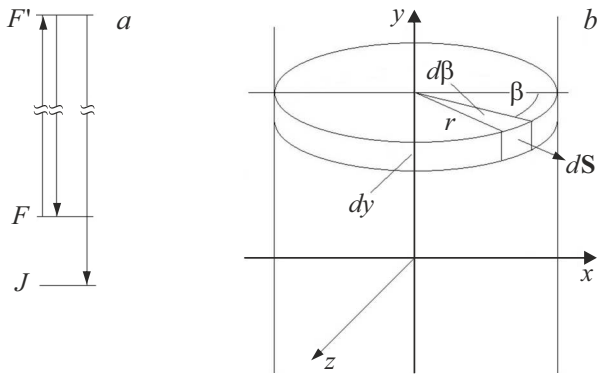
Рис. 3. а) Резонансные мультиплеты F (основной) и F' (возбужденный). Низходящими стрелками показан радиационный распад и сверхтонкая накачка нерезонансного мультиплета J . б) К вычислению энергии, поглощаемой скоростными группами из зондирующего пучка.
