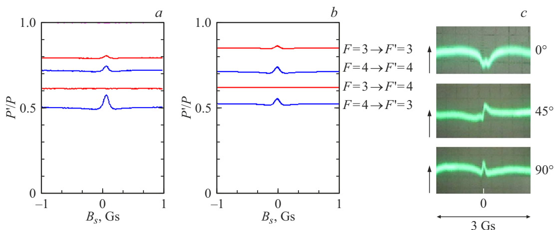
Рис. 2. Зависимость поглощения от магнитного поля в геометрии Фойхта для различных переходов линии D1 цезия a — эксперимент, b — теория. Зависимости a и b получены при угле между направлением линейной поляризации зондирующего пучка и магнитным полем соленоида 90^\circ . ( c ) Поведение поглощения P'/P на переходе F = 4 \rightarrow F' = 3 при прохождении поля соленоида через ноль для различных углов (углы показаны справа) между магнитным полем соленоида и направлением линейной поляризации зондирующего пучка.
