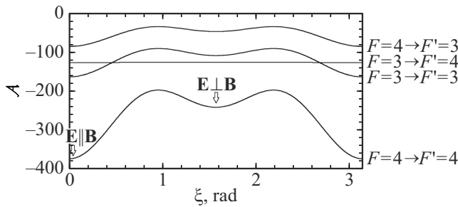
Рис. 4. Зависимость нелинейного вклада \mathcal{A} (35) в пропускание от угла \xi между магнитным полем и направлением линейной поляризации зондирующего пучка (36) для всех переходов линии D1 цезия. Видно, что в соответствии с экспериментом развитая теория показывает фактически полную изотропию перехода F = 3 \rightarrow F' = 4 .
